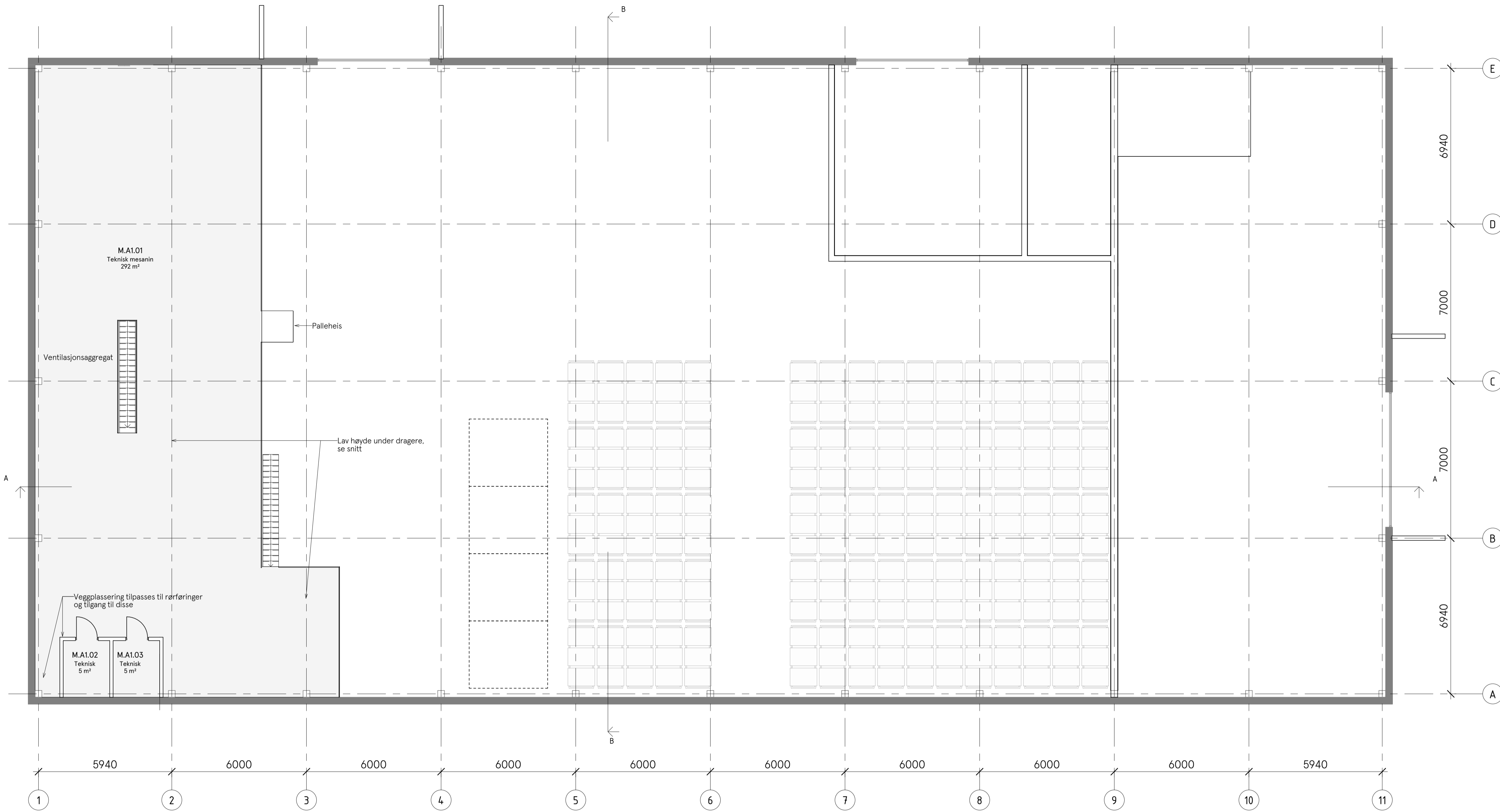
Plan mesanin 1 : 100
