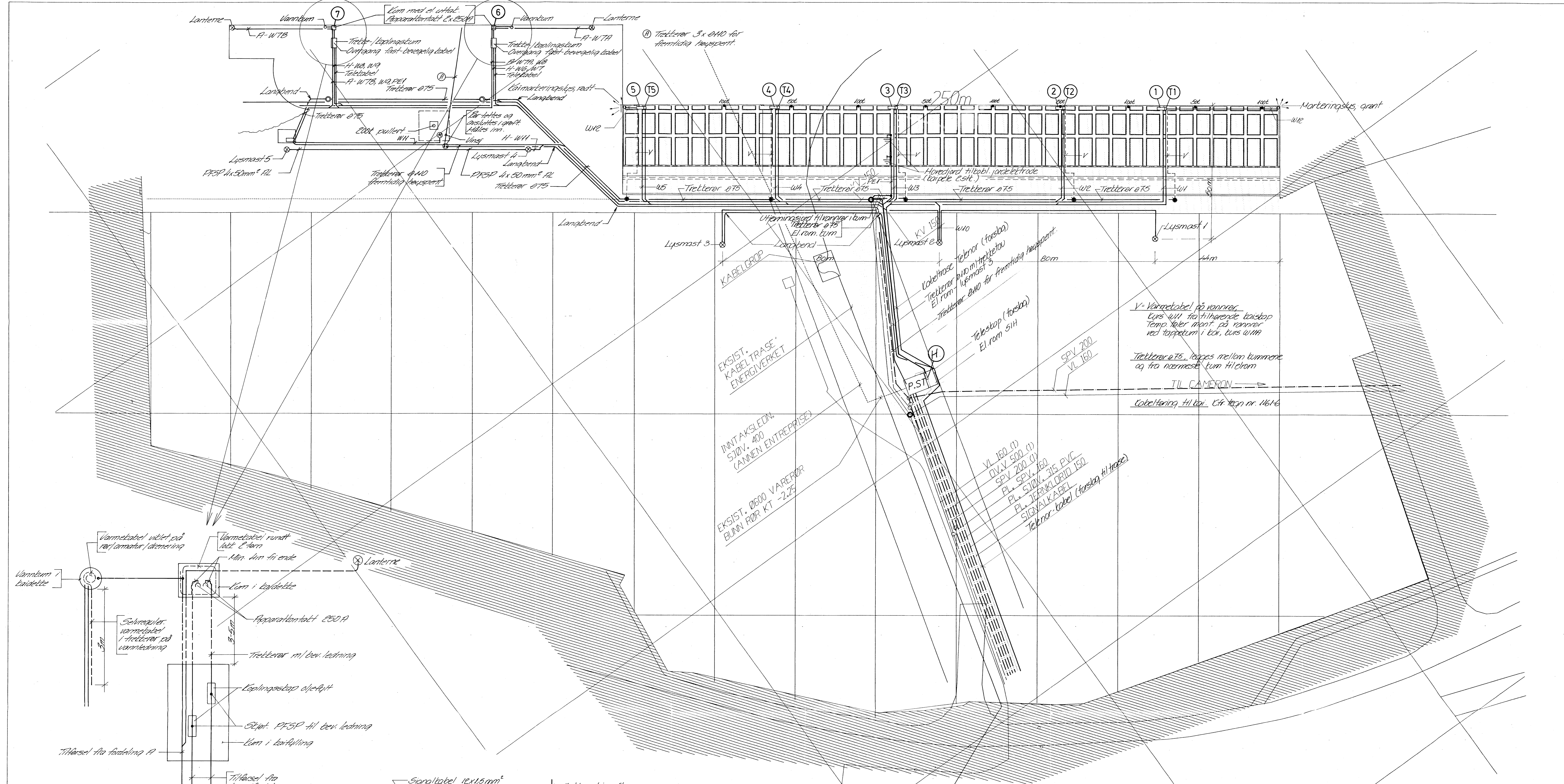
Prinsipp installasjon kai
