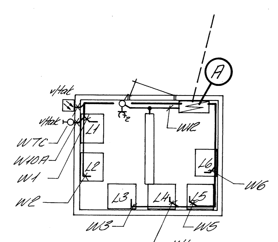
Bygg for antiferrosprosianlegg Mål 1:50
