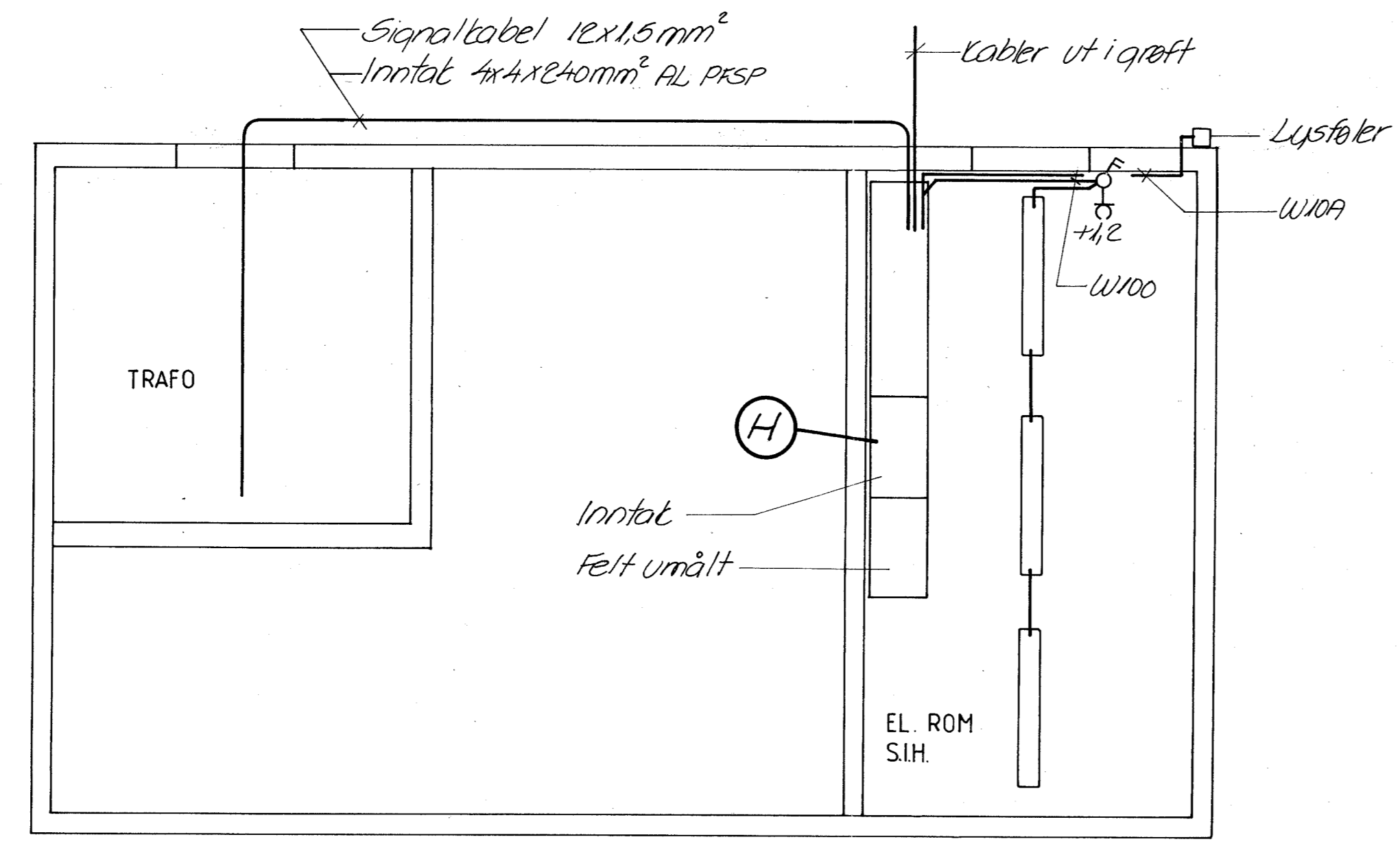
Mål 1:50 El installasjoner i el rom
