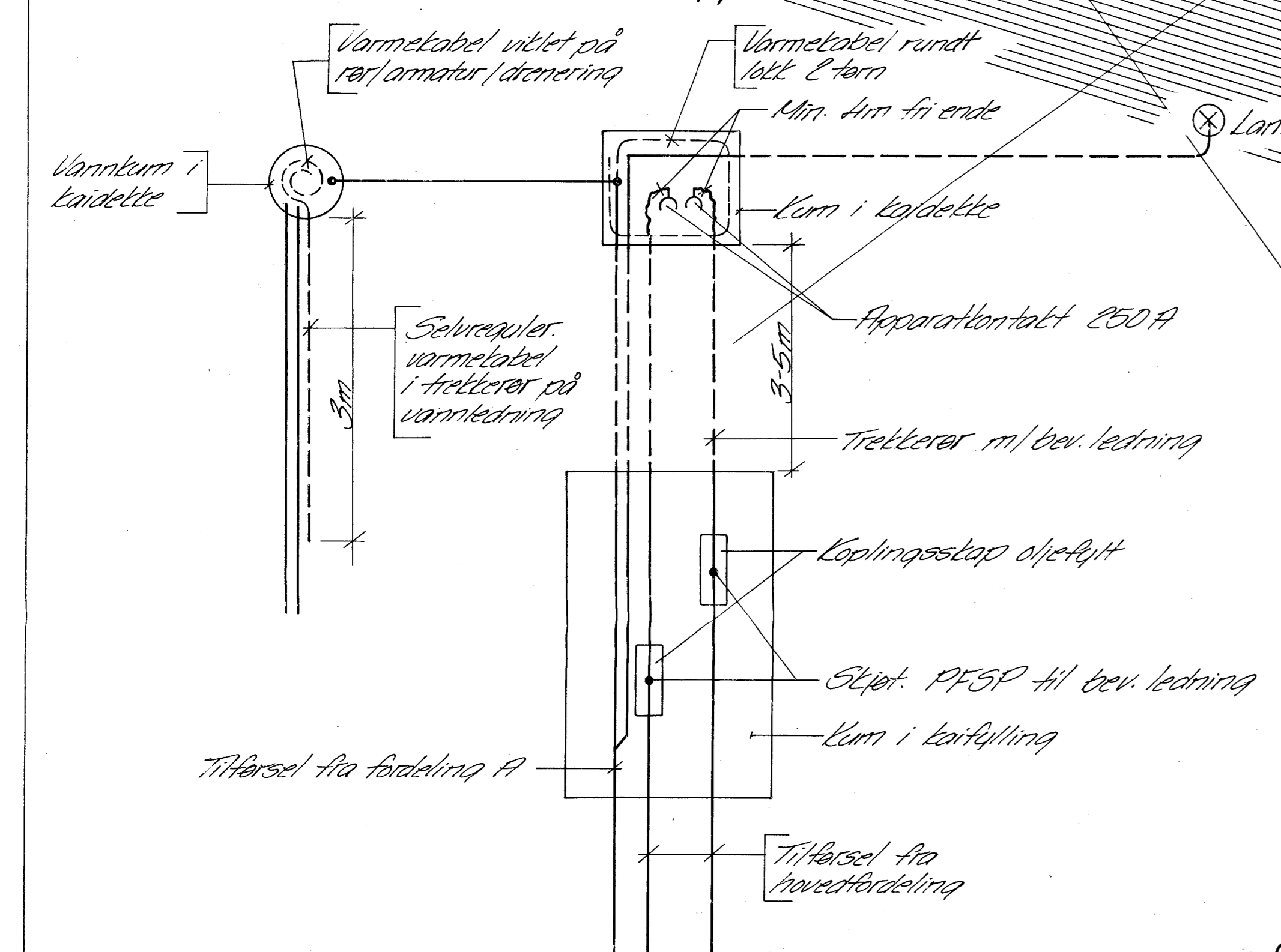
Prinsipp installasjon kai
