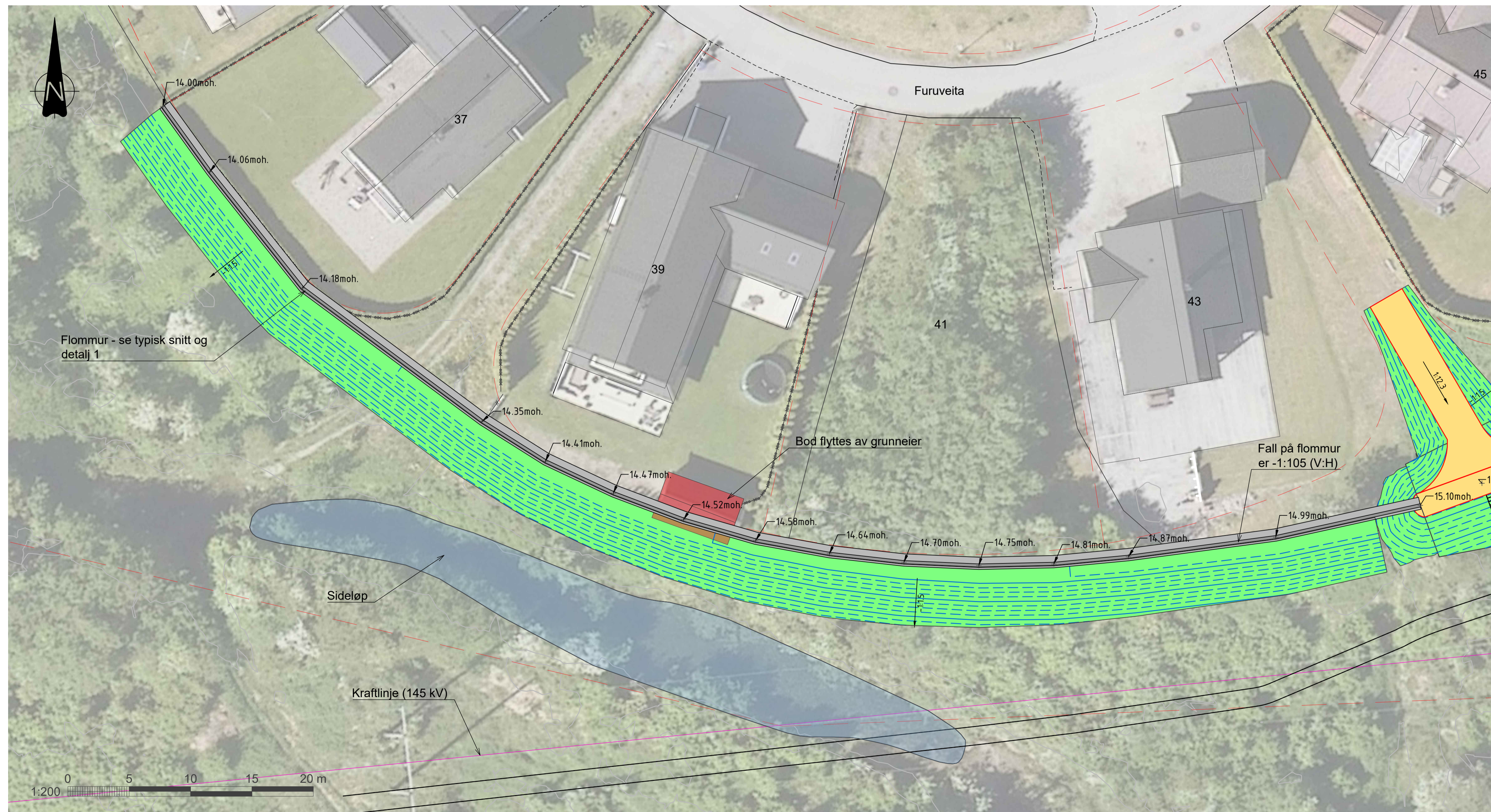
OVERSIKT - FLOMMUR 1:200 m
