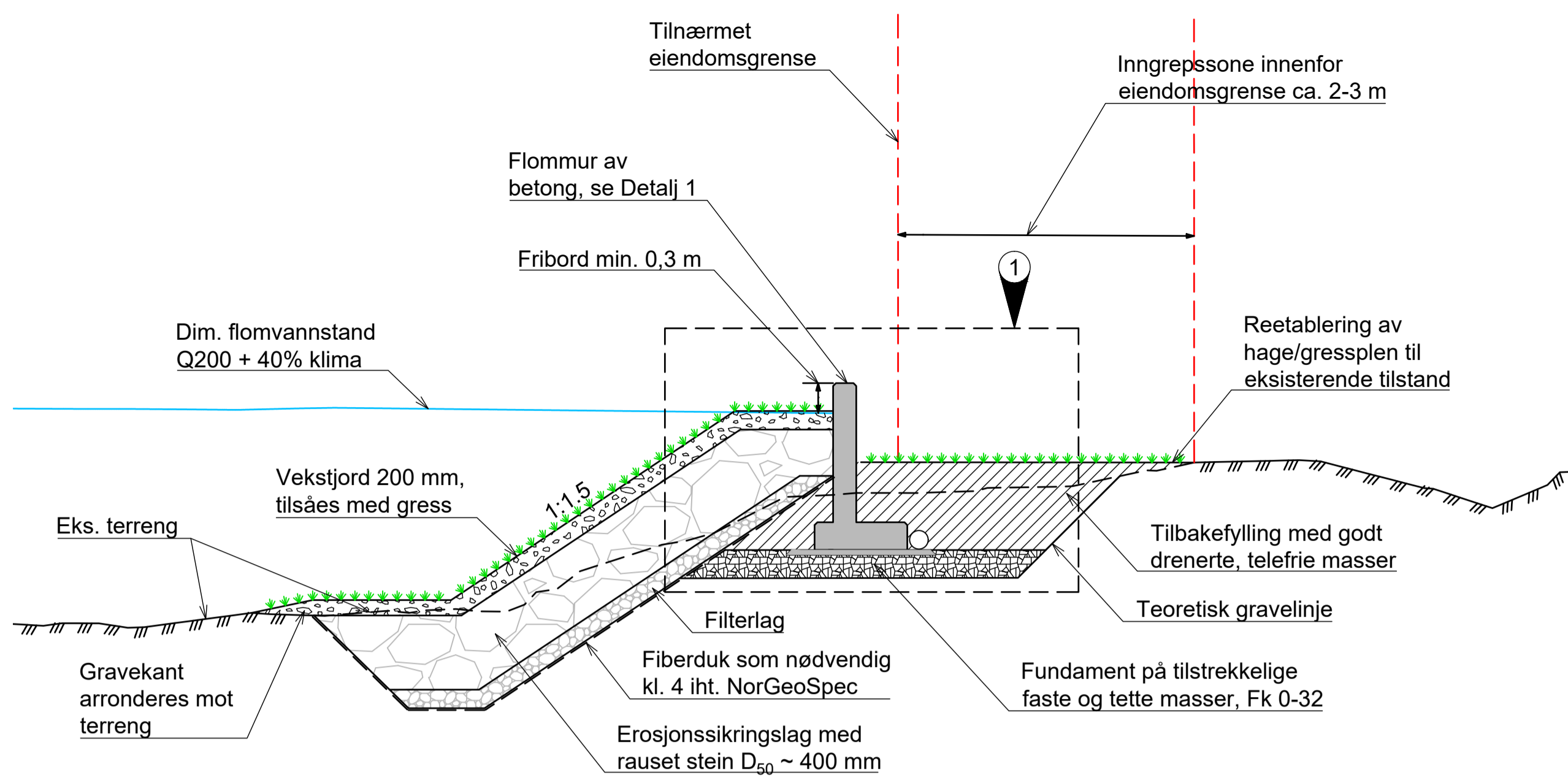
TYPISK SNITT - FLOMMUR AV BETONG 1:50 m
