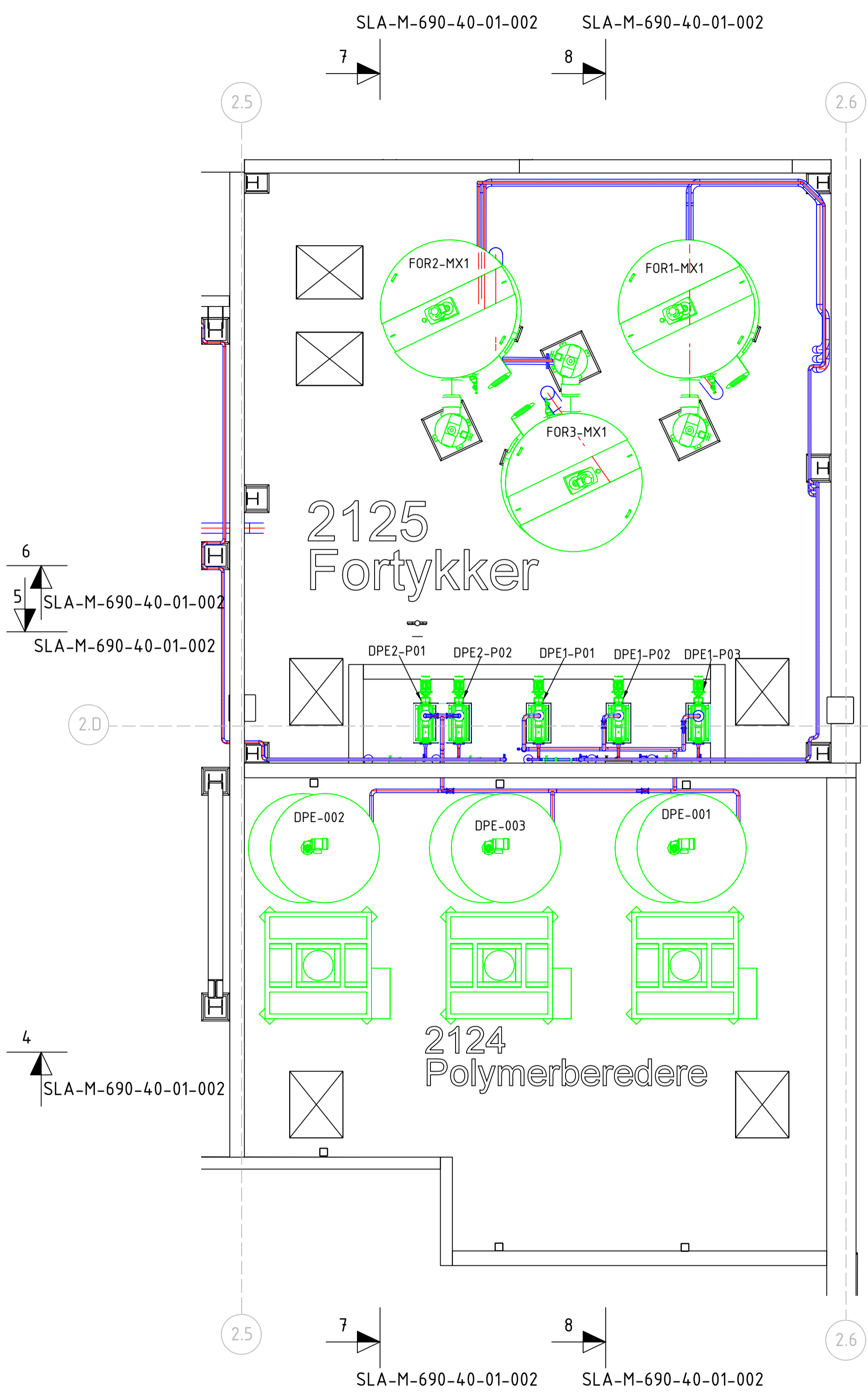
Plan 1 - Fortykkere og polymer-rom 1:50
