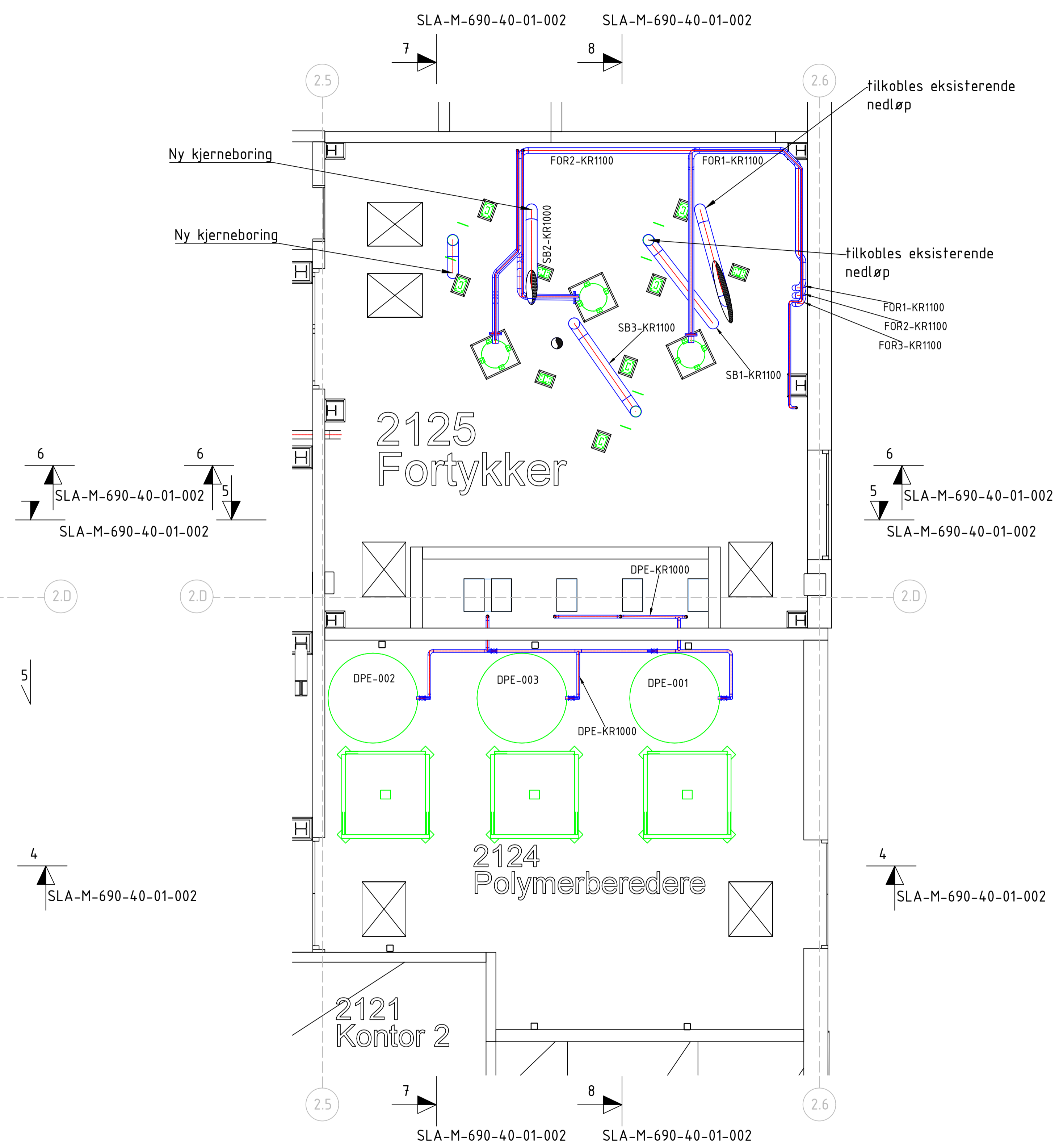
Plan 1 - Fortykkere og polymer-rom k+1.0 1:50
