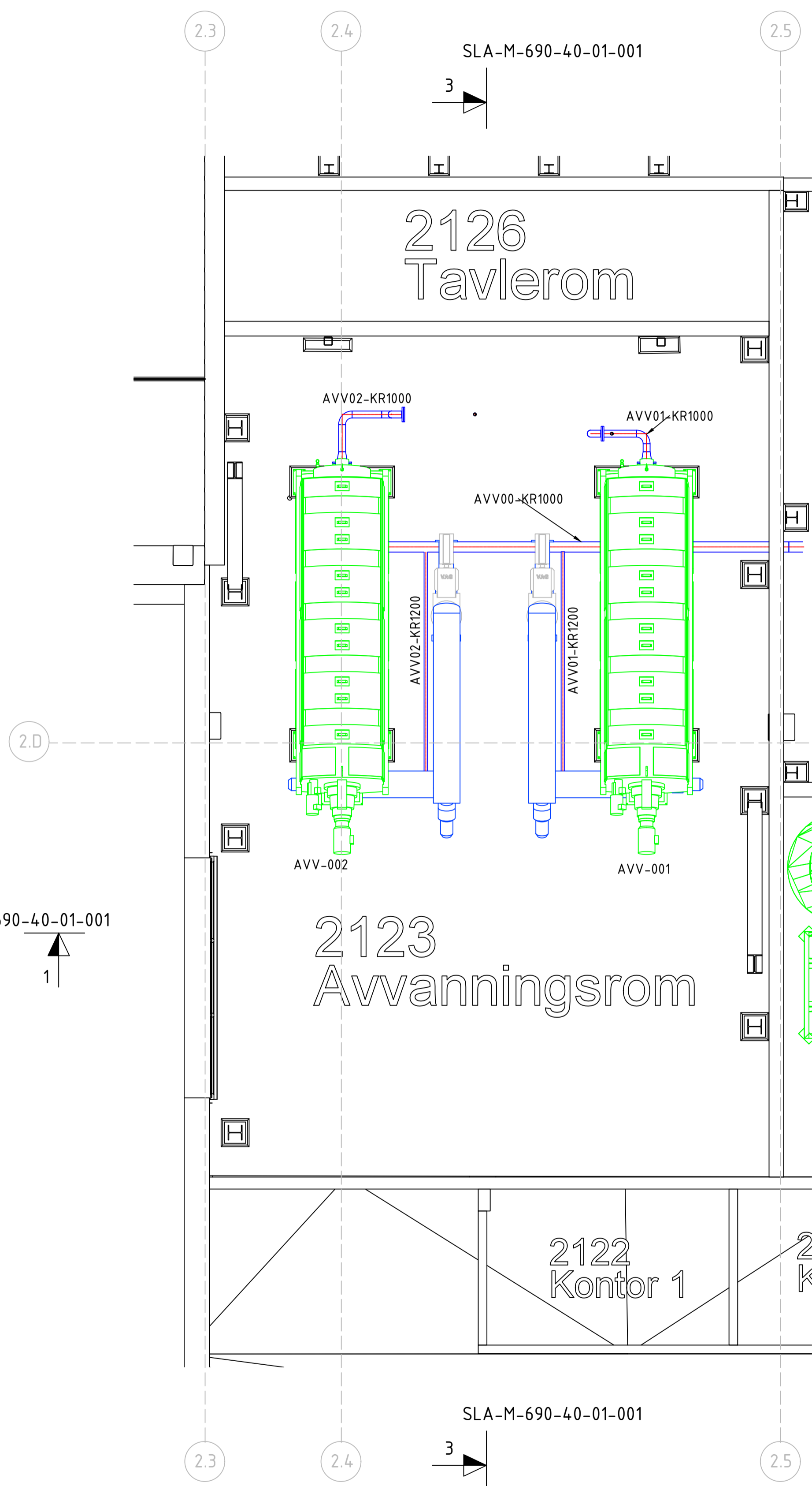
Plan 1 - Avvanningsrom 1:50
