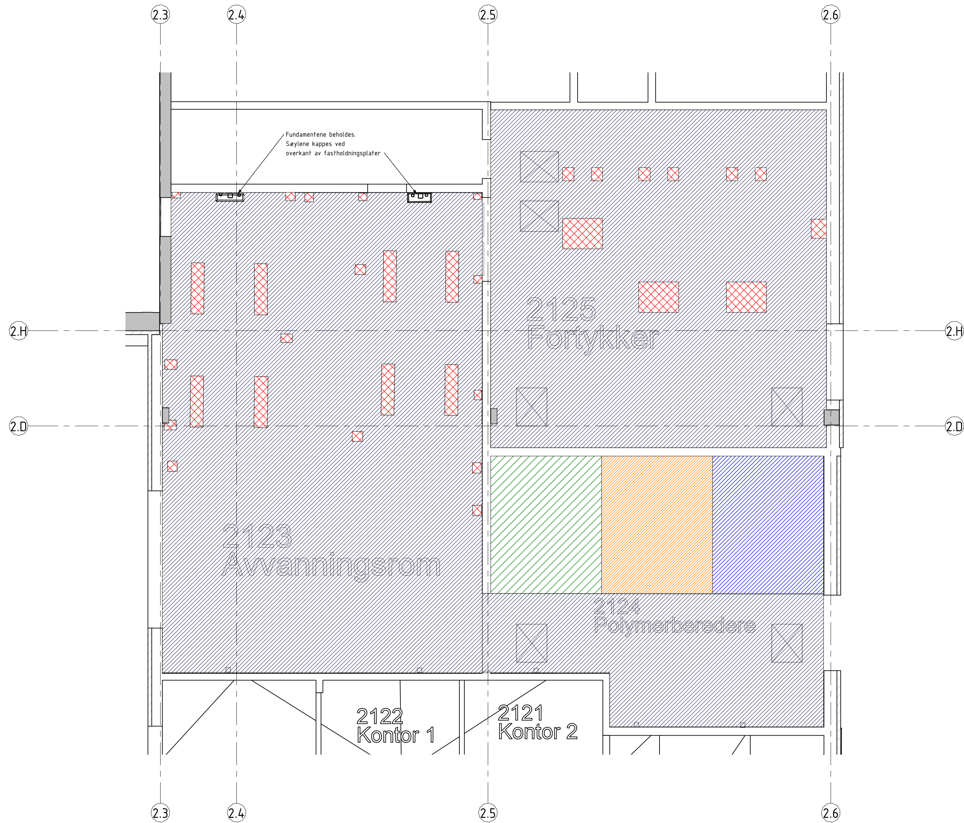
1 Rivetegning Avvanningsrom, Fortykkerrom og Polymerrom Plan 1 : 50
