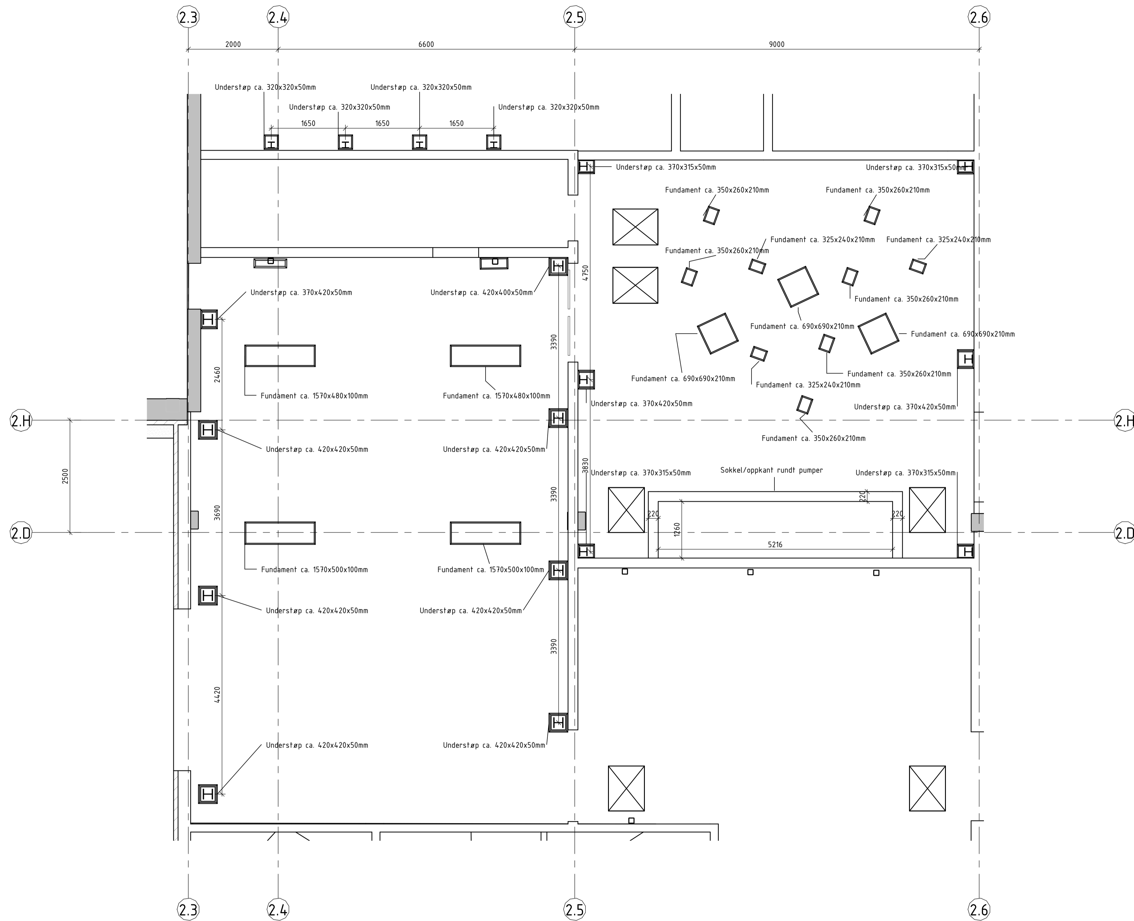
Nye fundamenter, understøper og sokkel i Avvanningsrom og Fortykkerrrom 1:50
