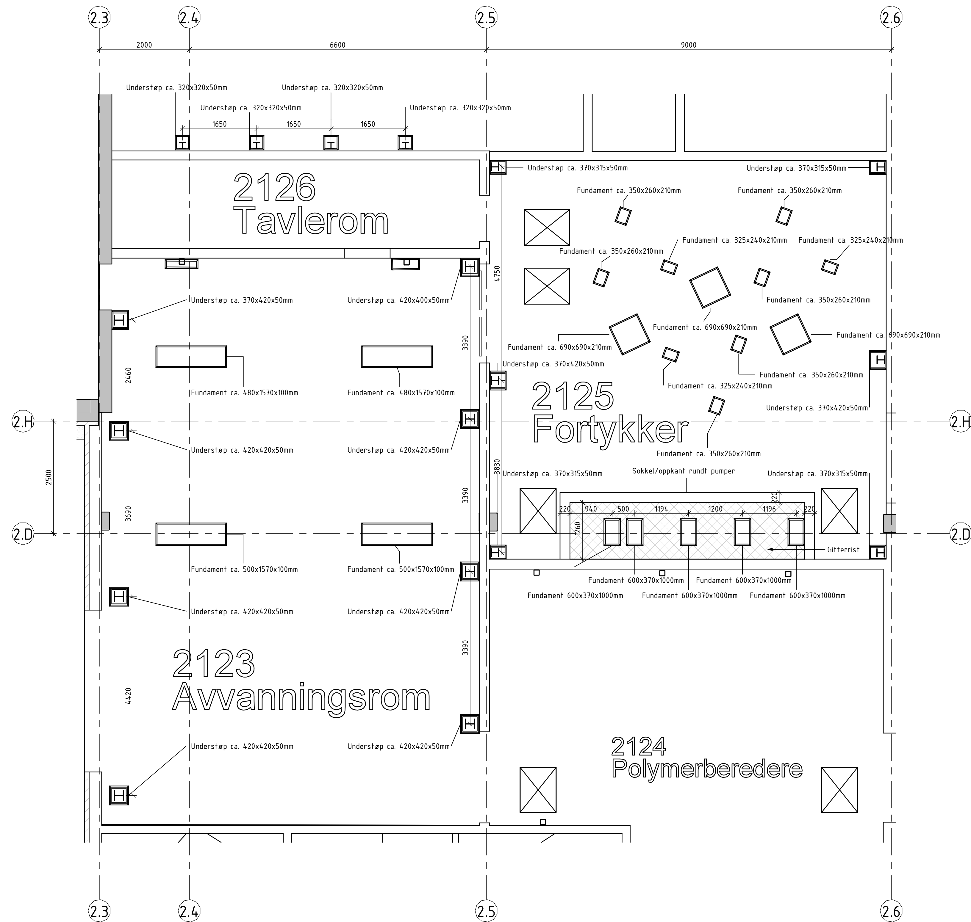
Nye fundamenter, sokler og understøper 1 : 50
