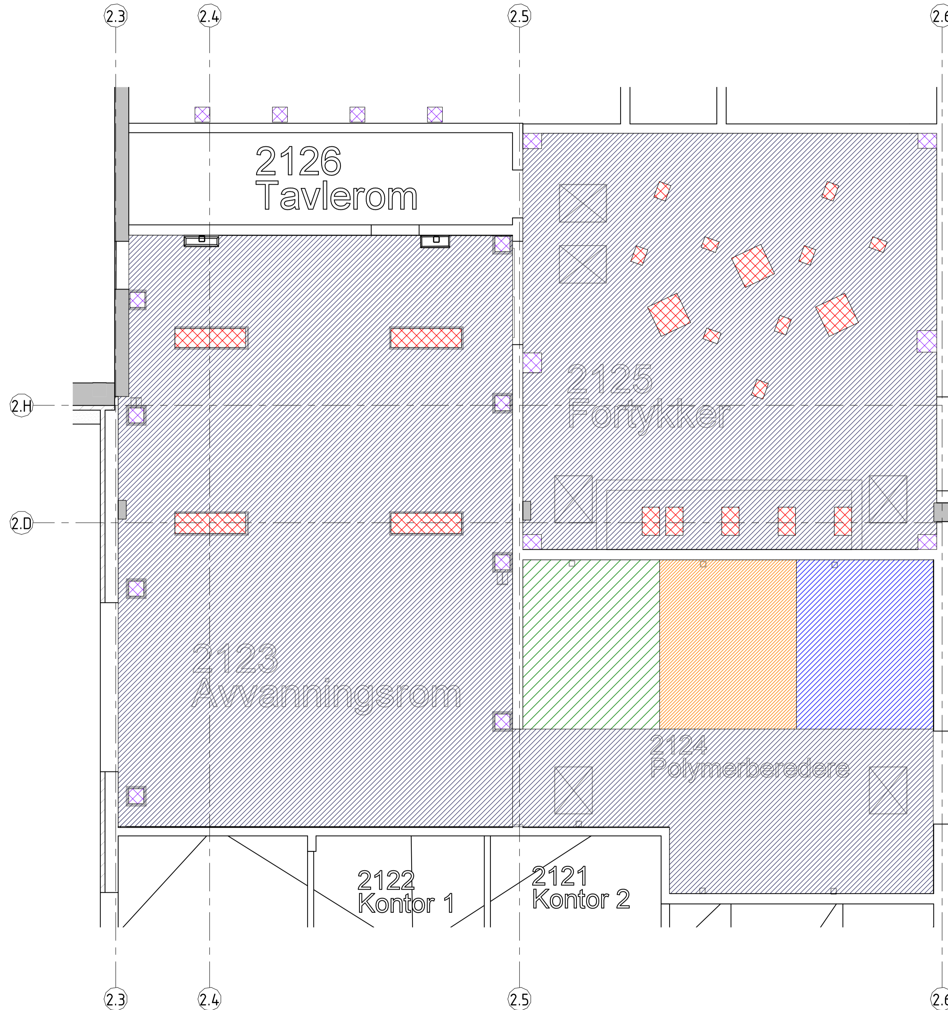
Nytt belegg og fundamenter 1 : 50
