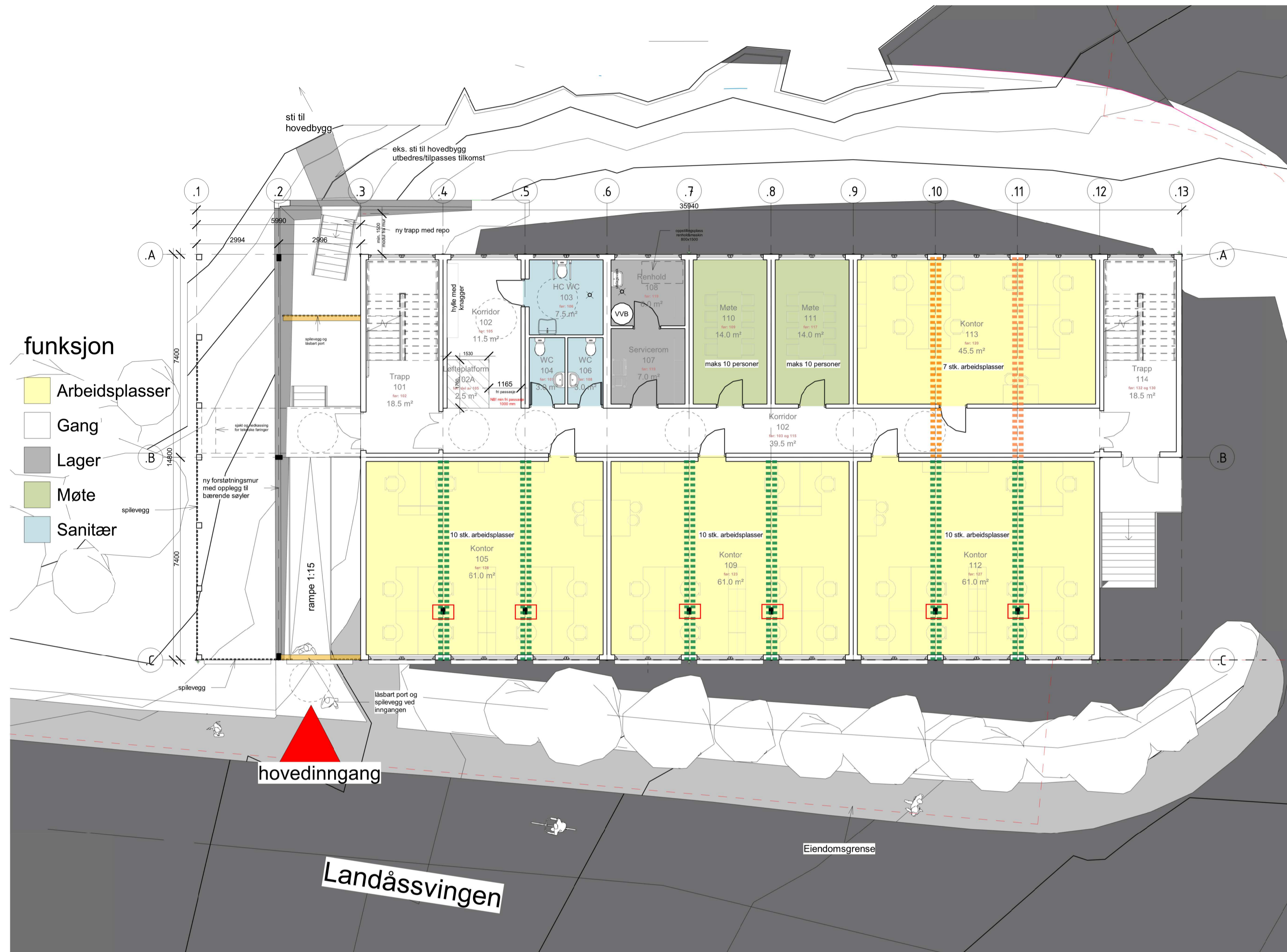
Modulbygg Plan 01 1 : 100
