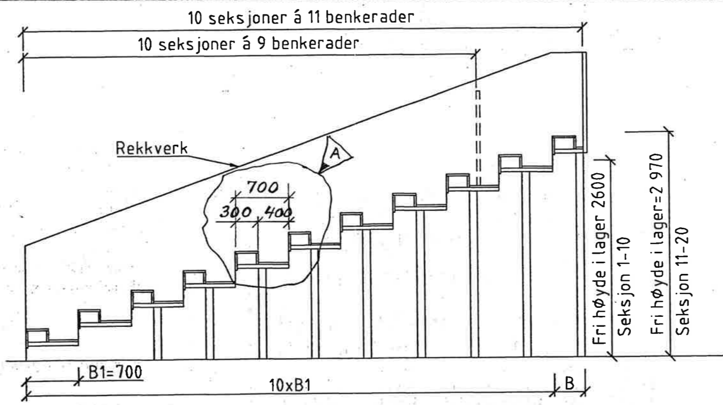
Prinsipptegning. Snitt teleskoptribune 1:50
