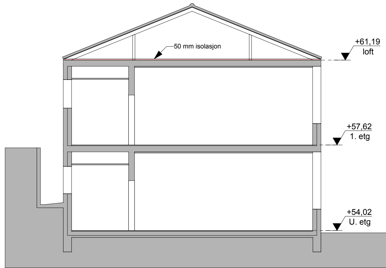
SNITT FØR TILTAKET.
