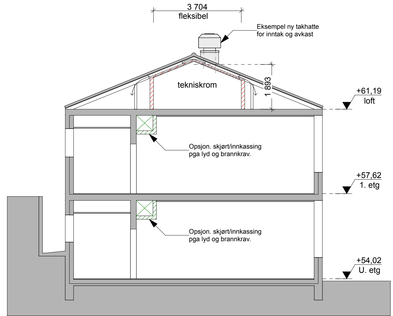
SNITT ETTER TILTAKET.
