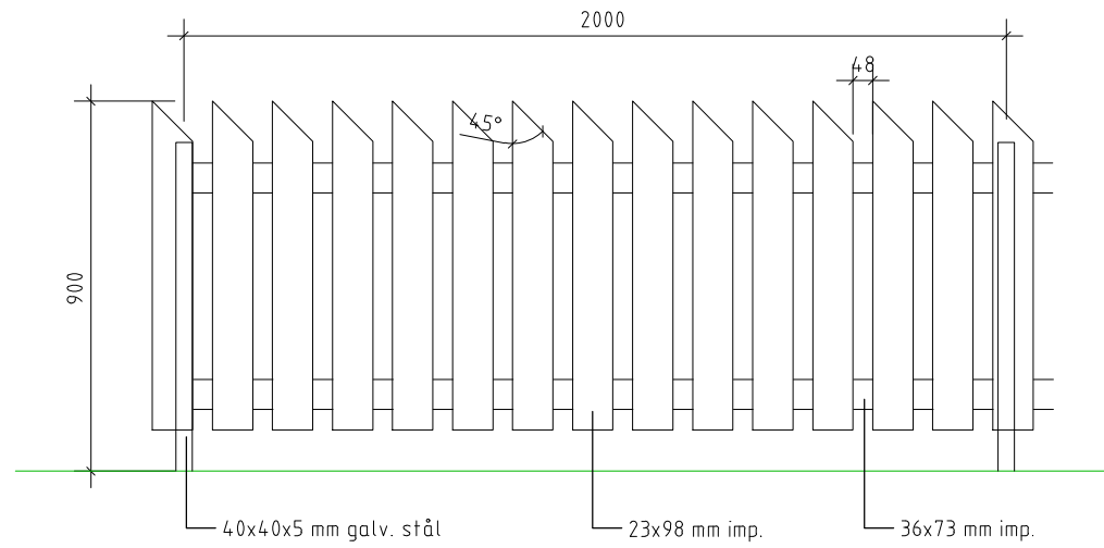
Oppriss gjerde alternativ 1 (gjelder arbeidsavsnitt 2 og 3) M=1:10
