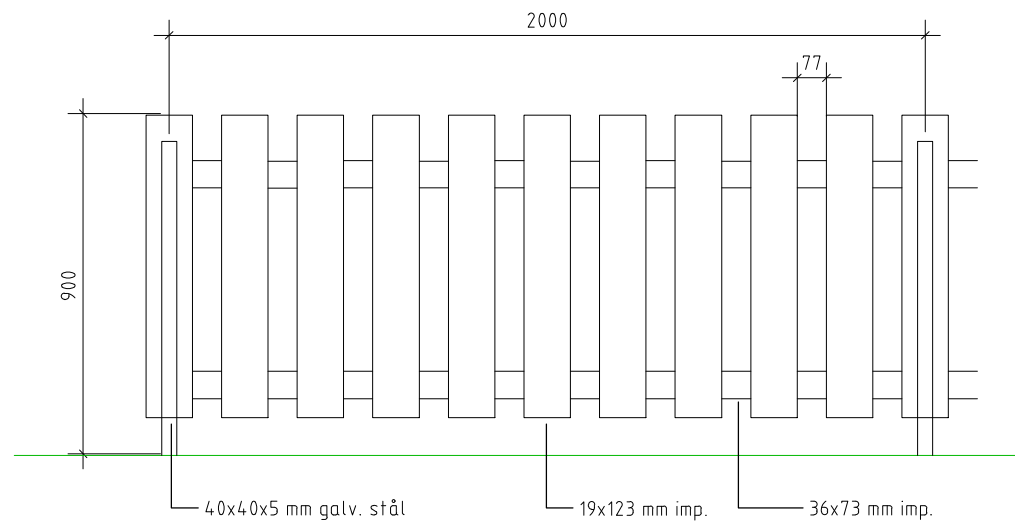
Oppriss gjerde alternativ 2 (gjelder arbeidsavsnitt 2 og 3) M=1:10
