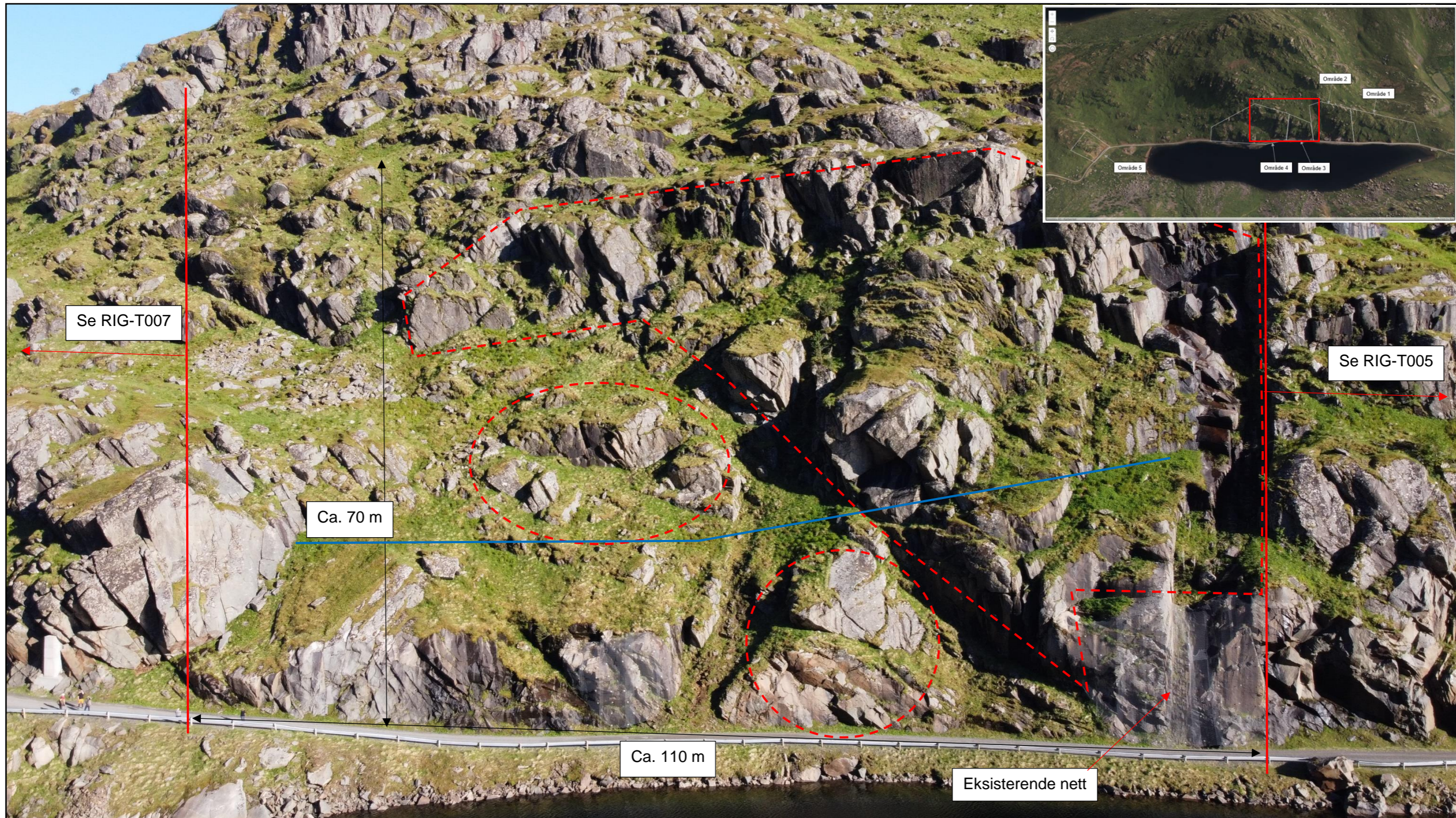
Område 4. Røde stiplede linjer viser omfang av rensk. I tillegg blir det behov for bolter og/eller stag. Eksisterende nett må forsterkes med bolter. Blå strek indikerer plassering av evnt fanggjerd
