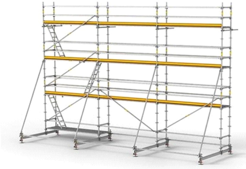
Systemstillas med rekkverk, avstivere, sparkelist og støtteben.
