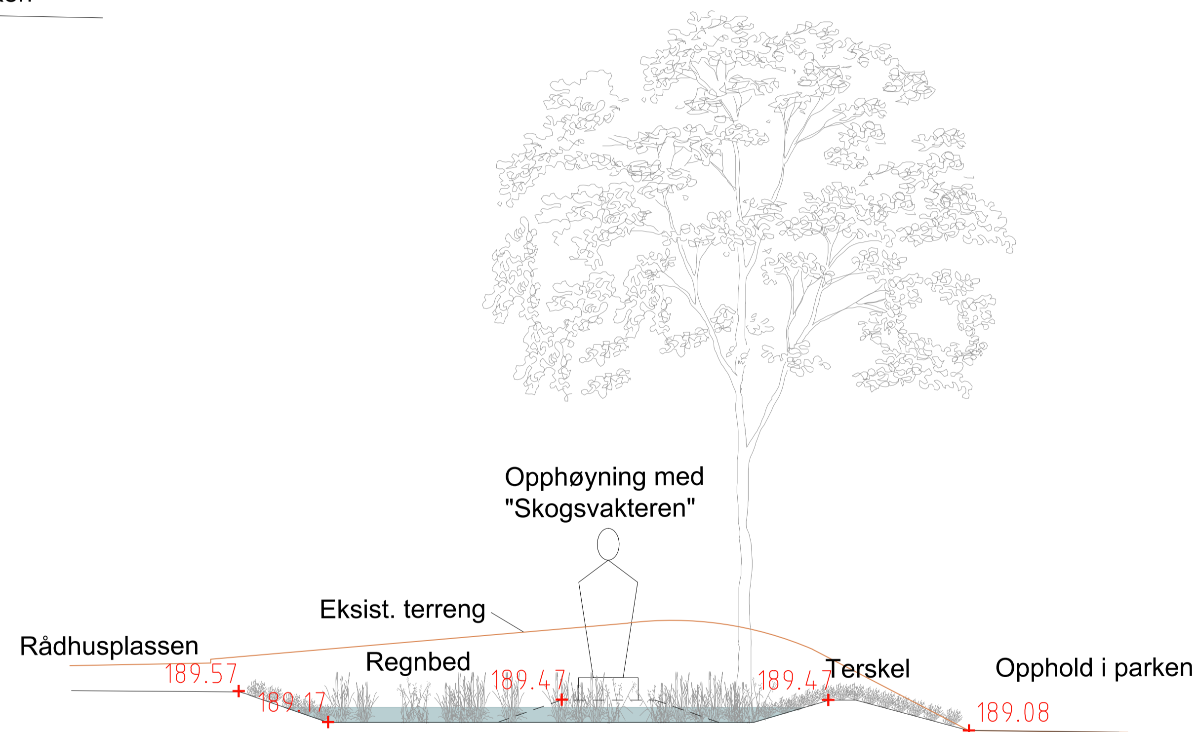
Snitt B-B' M. 1:50
