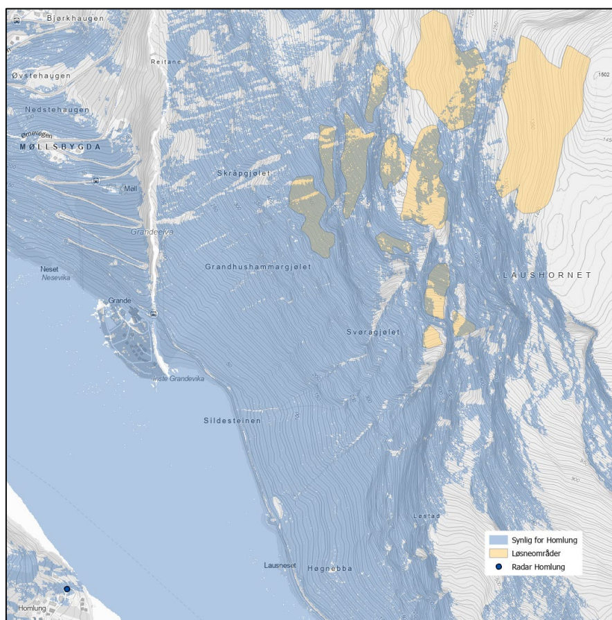
Figur 5 Resultat av siktanalyse fra Homlung. Sikt fra radarplassering er markert som blå skravur og løsneområder som oransje polygon.
