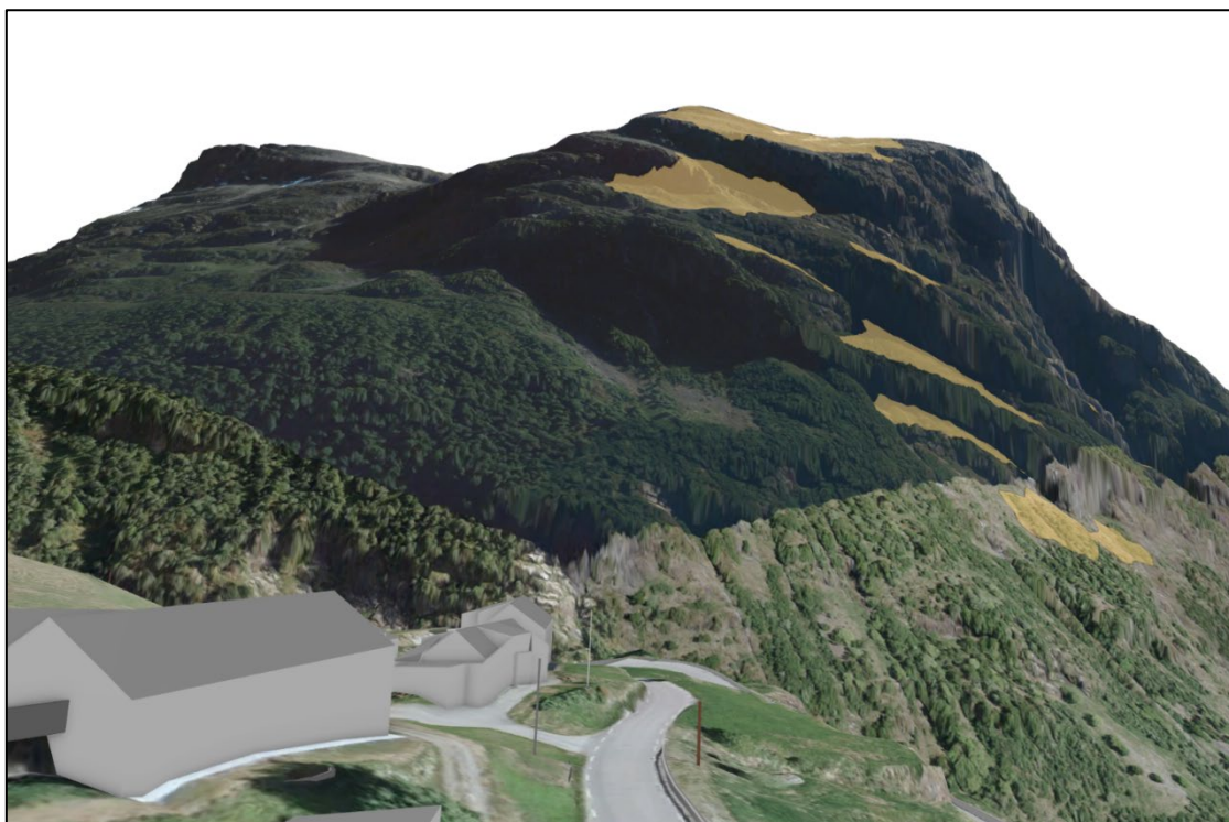
Figur 4 Utsyn fra radarplassering på Møllsæter, løsneområdene er vist som oransje polygon.
