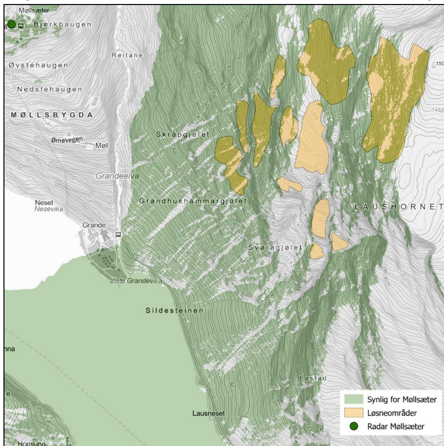
Figur 3 Resultat av siktanalyse fra radarplasseringen på Møllsæter. Sikt fra radarplassering er markert som grønn skravur og løsneområder som oransje polygon.
