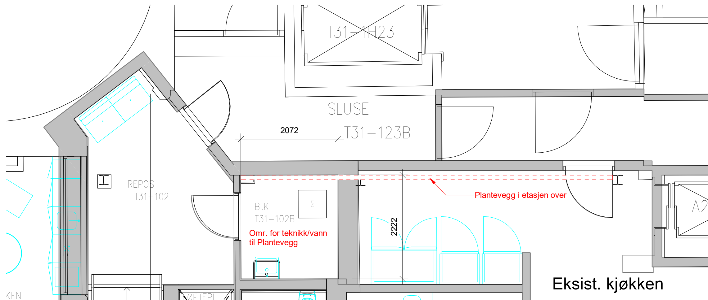
Plan 1 et. M:1:50
