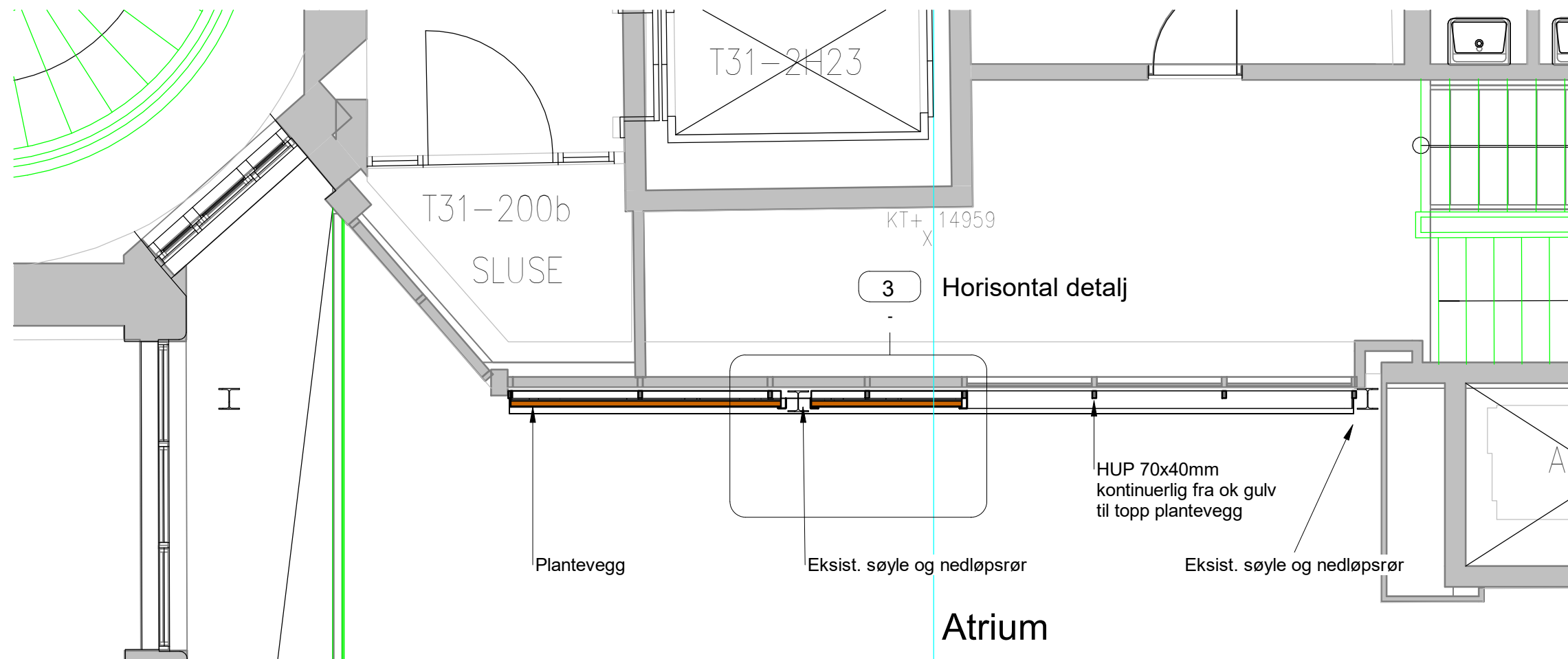
Plan 2 et. M:1:50
