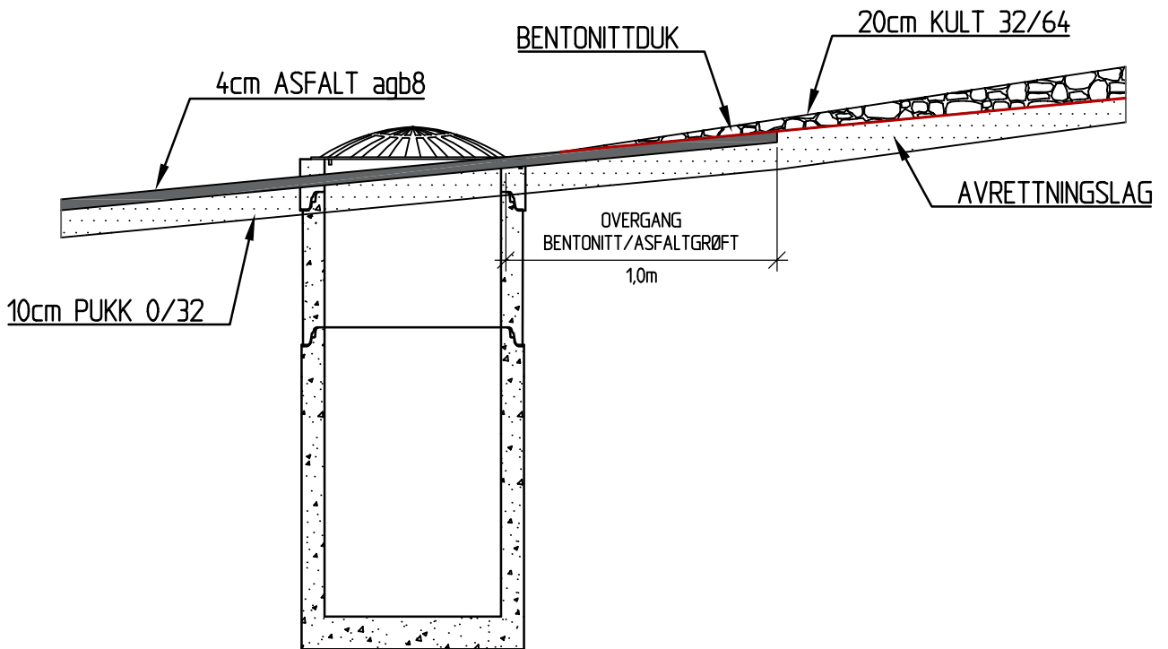
SNITT A-A:
