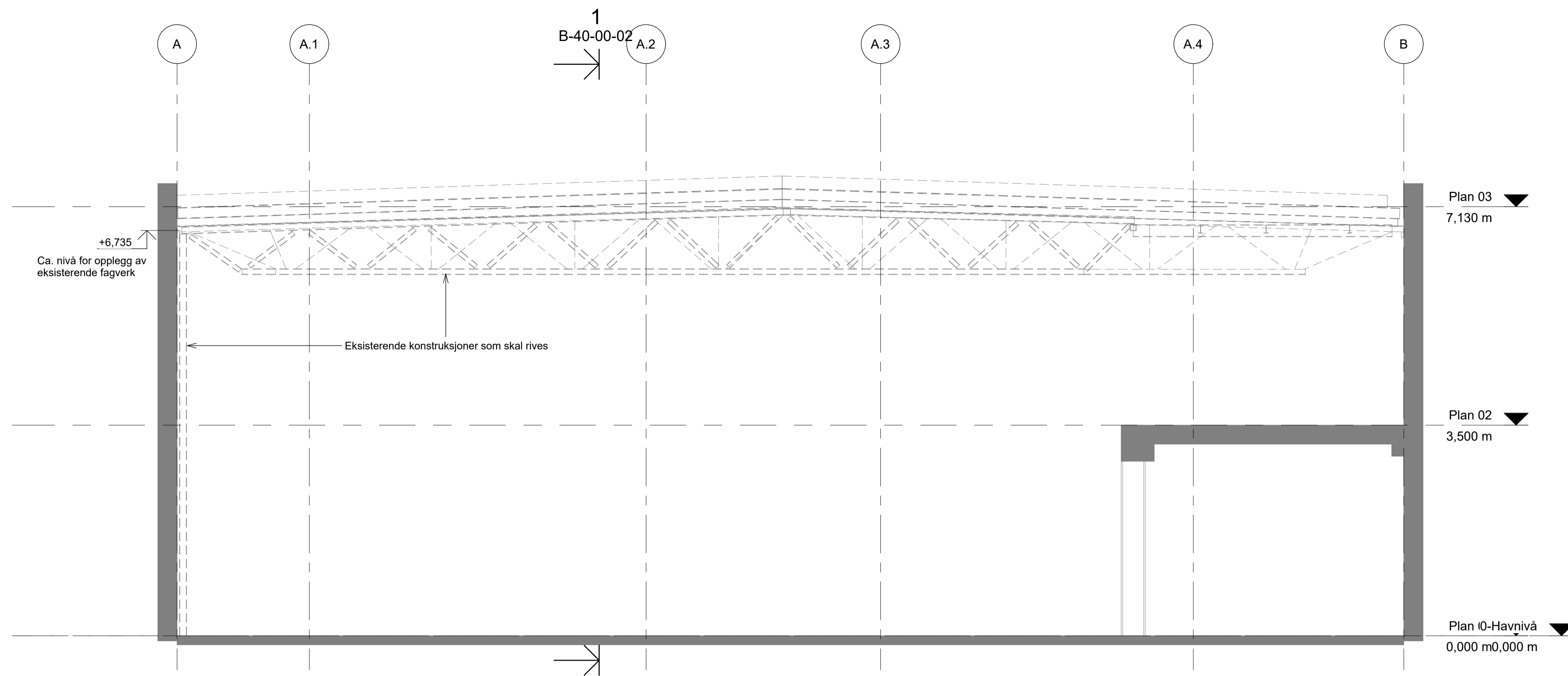
1 EKSISTERENDE KONSTRUKSJONER 1 : 50
