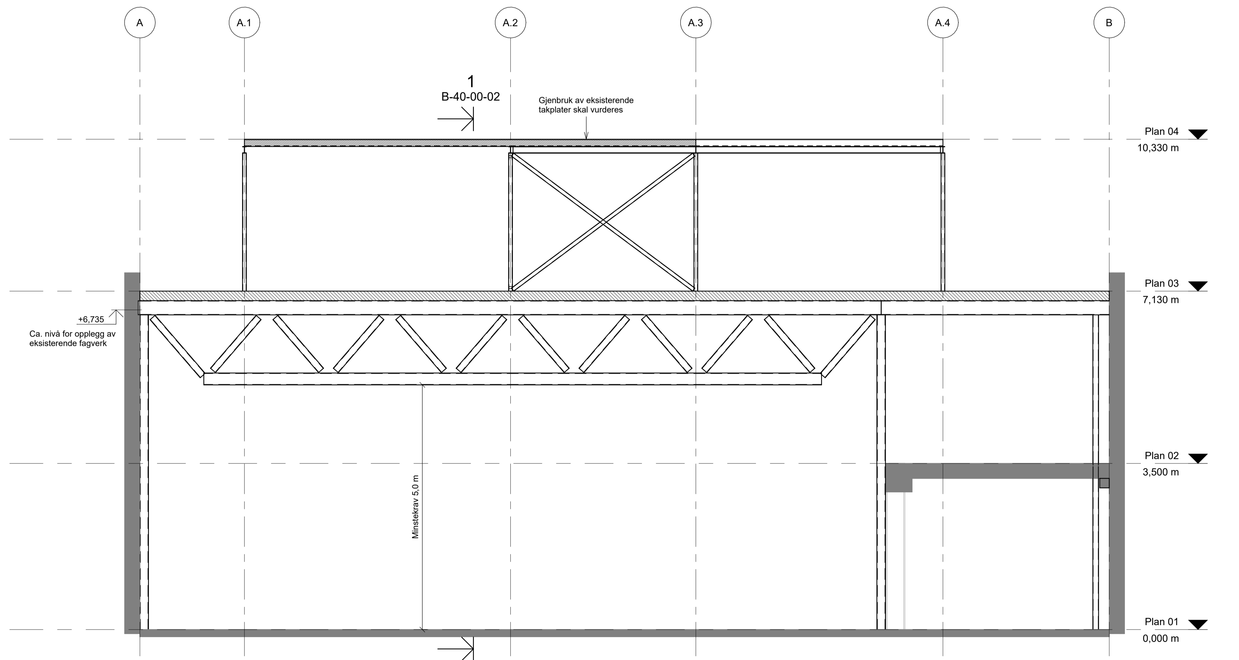
2 OMBYGGING 1 : 50
