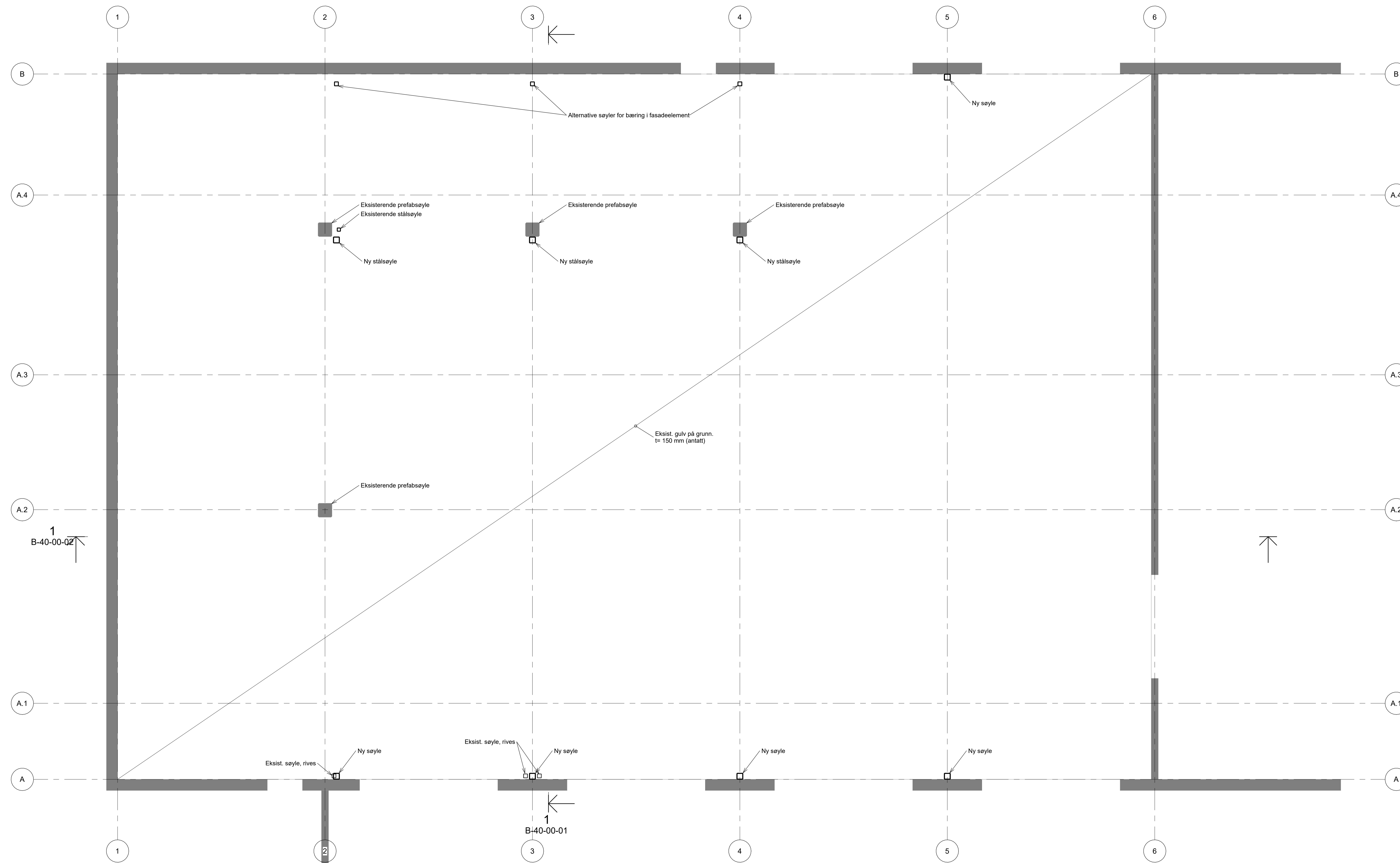
PLAN 1. ETASJE, OMBYGGING 1 : 50
