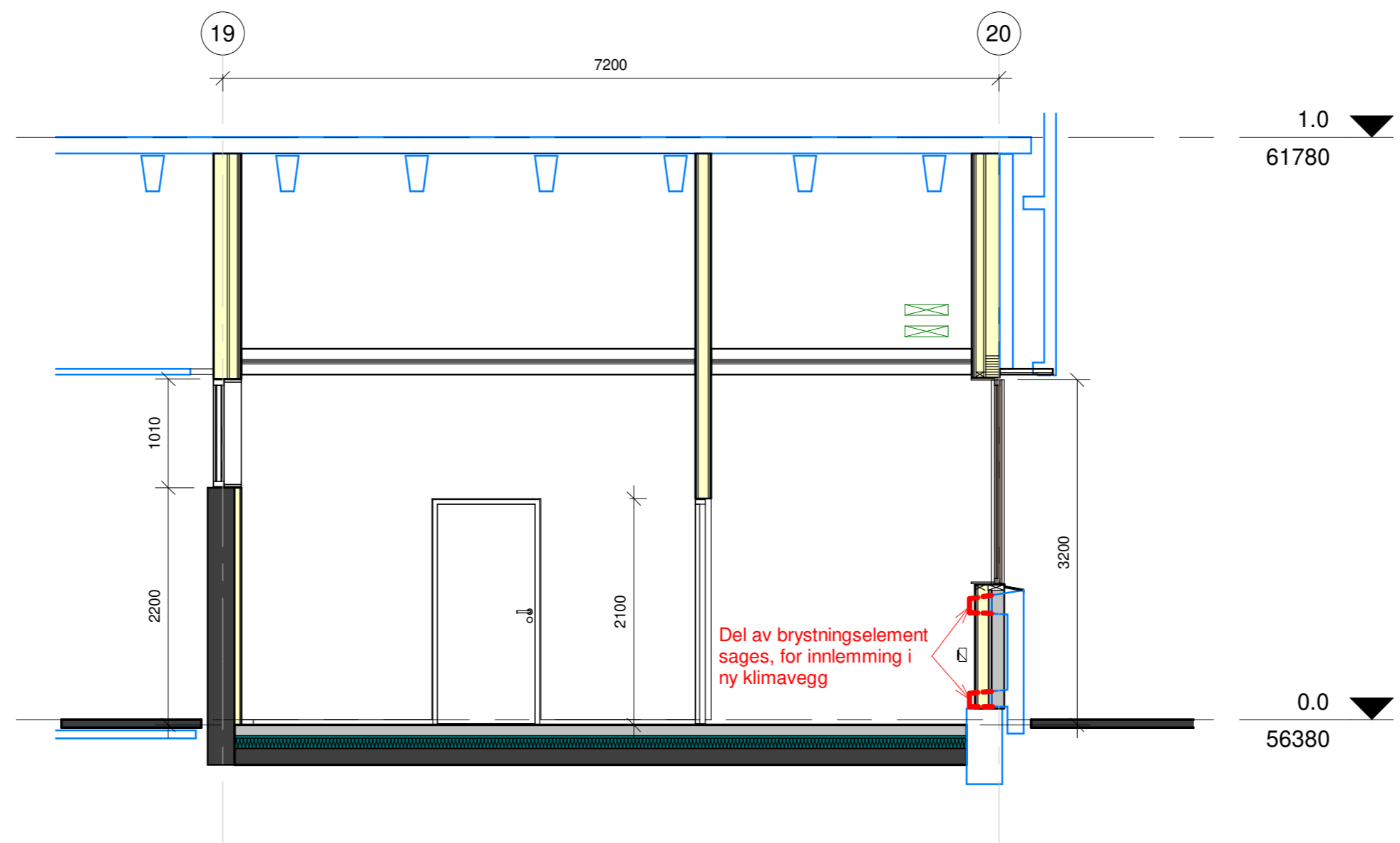
3 Snitt A 1 : 50
