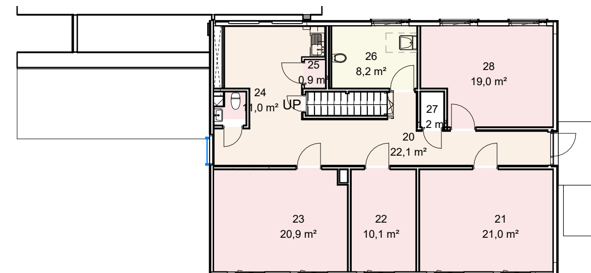
1 1 etasje Paviljon 7 Rombehandling 1 : 150
