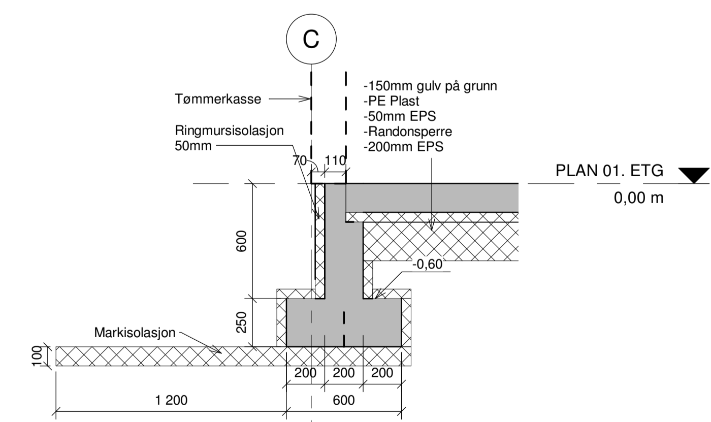
S1-Bankett-ringmur 1 : 20
