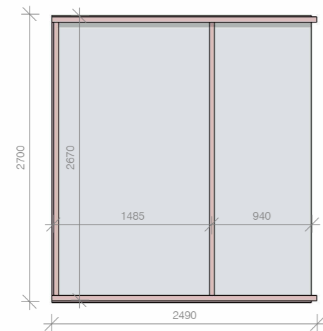
61 002-2 Glassfasade vest 1 : 50
