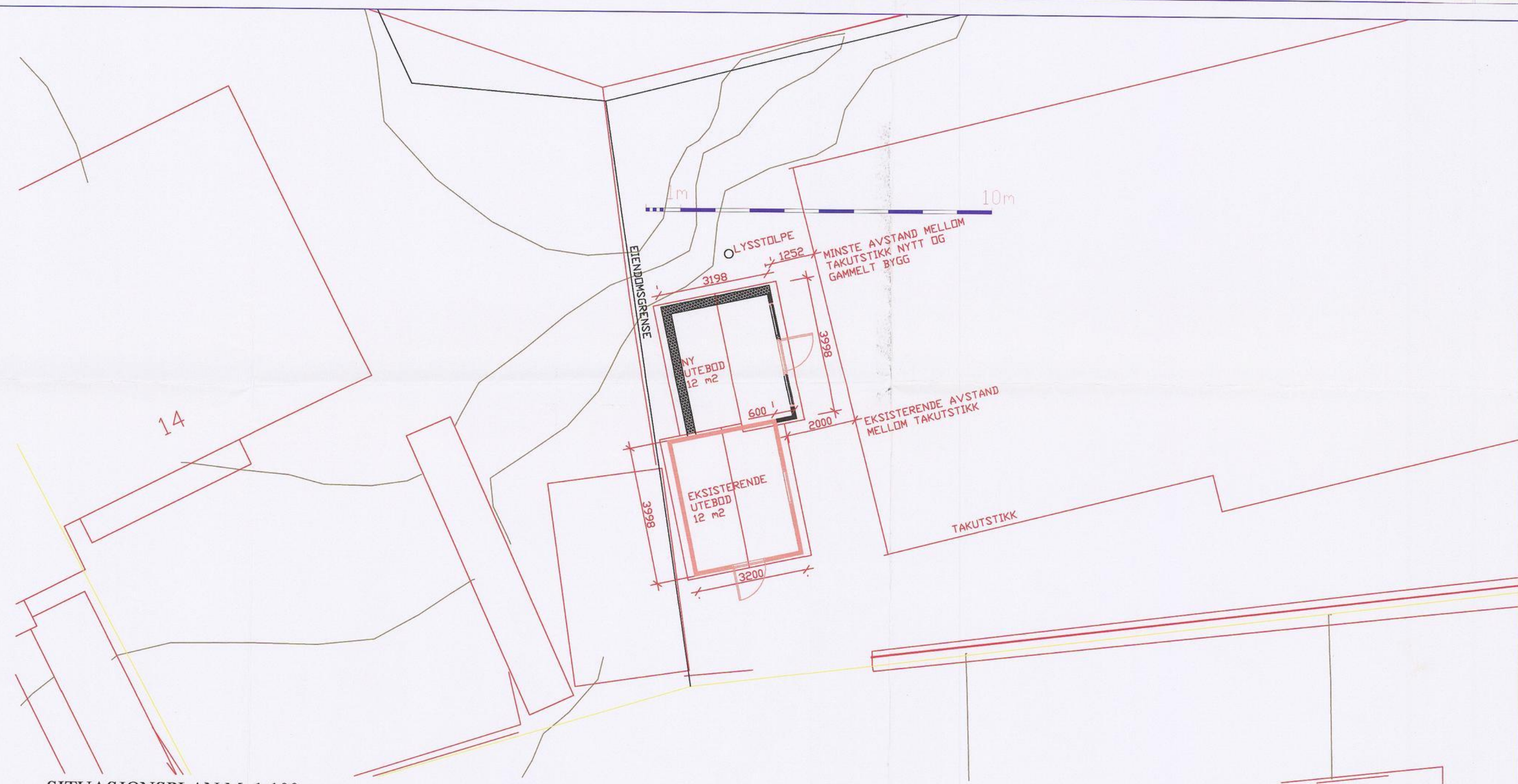
SITUASJONSPLAN M=1:100
