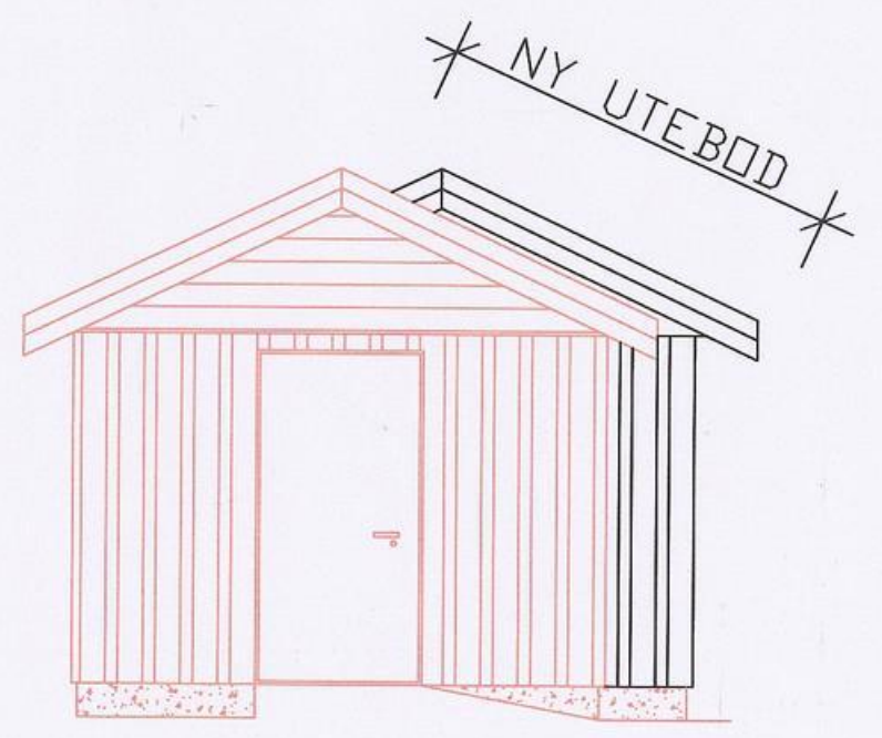
FASADE SØR 1:50
