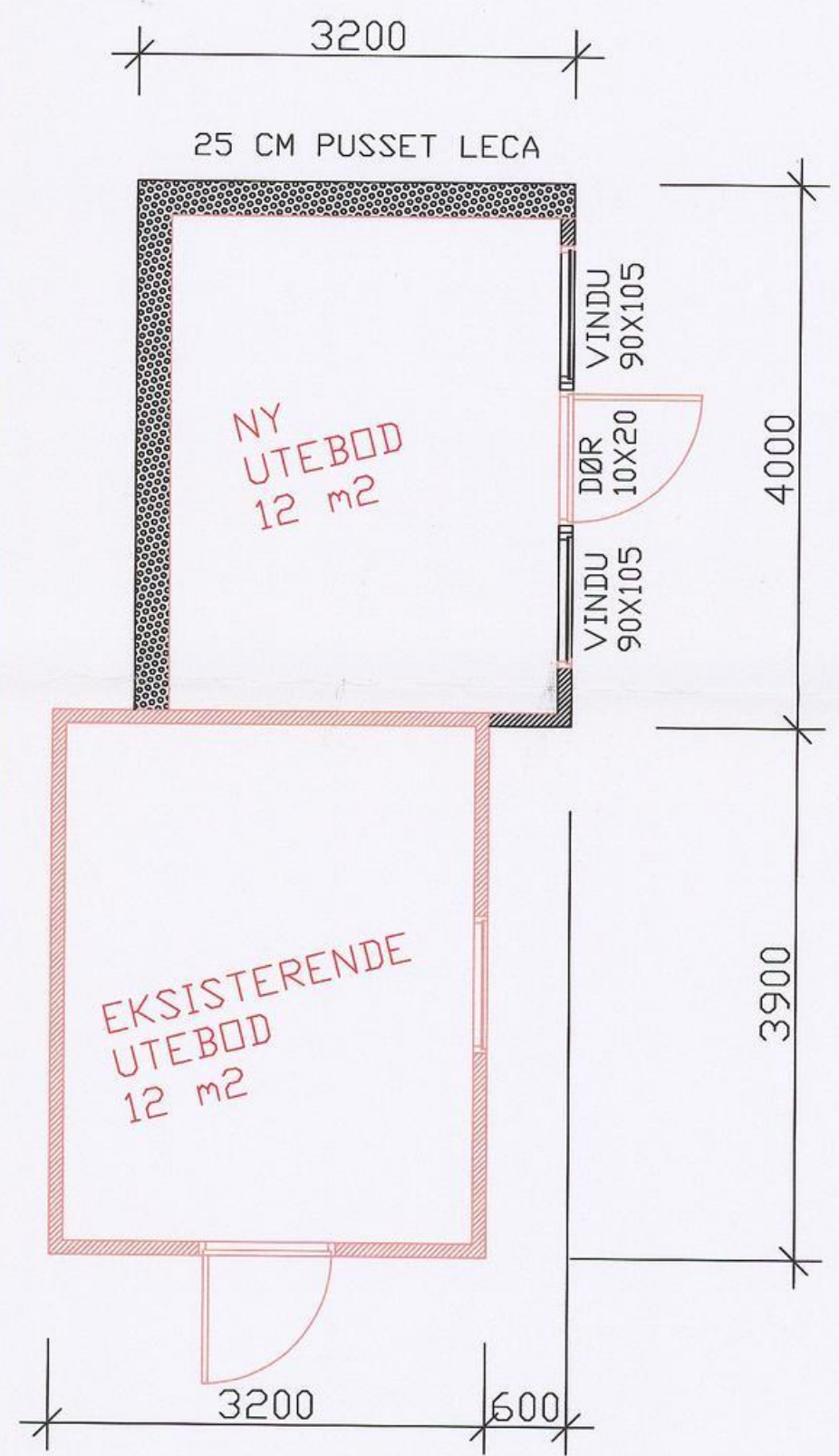
PLAN UTEBODER 1:50
