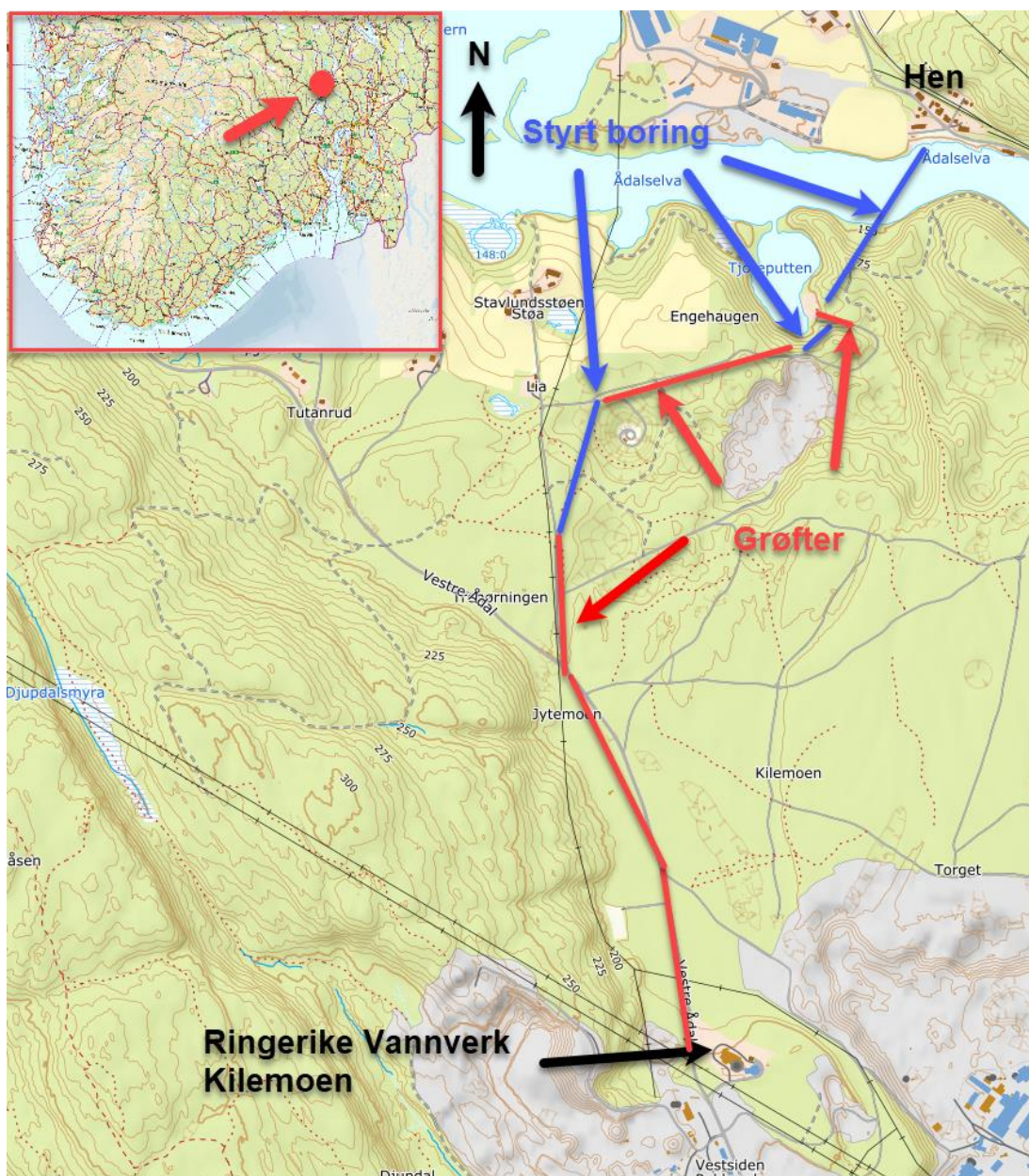
Figur 1: Oversiktskart over planlagt tiltak. Det skal legges 2 vannledninger (Ø500 og Ø315) fra Ringerike Vannverk Kilemoen til Tjoreputten. Fra Tjoreputten bores én vannledning (Ø315) videre under Ådalselva (styrt boring). Det benyttes grøftegraving og styrt boring på 3 avsnitt av traséen. Kilde: Norgeskart.no
