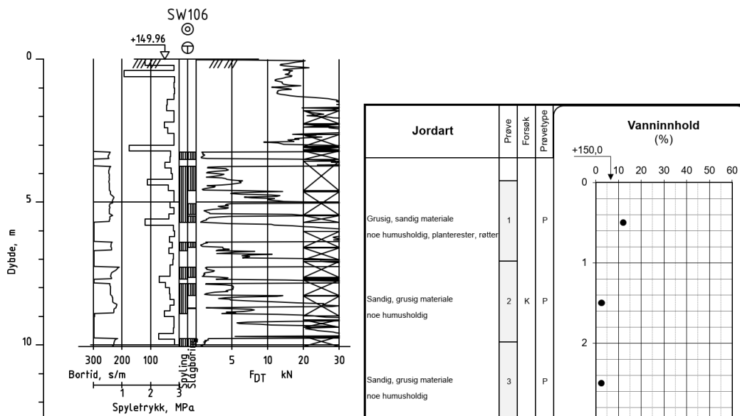
Figur 8: T.v.: Totalsonderingsprofil SW106, ca. ved pumpestasjon Tjoreputten som viser høy sonderingsmotstand og tyder stort sett på forekomst av sandig grusig materiale hele veien. T.h.: Utklipp som viser resultater fra prøvetaking SW106. Kilde: Datarapport [1]
