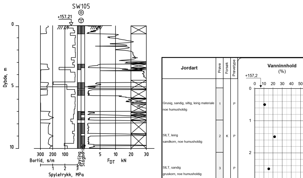
Figur 7: T.v.: Totalsonderingsprofil SW105, ca. ved pel 2050/VK6 som viser høy sonderingsmotstand og tyder stort sett på forekomst av sandig grusig materiale hele veien, men tyder på noen tynne, svakere lag mellom ca. 1 og 3 m. T.h.: Utklipp som viser resultater fra prøvetaking SW105. Kilde: Datarapport [1]
