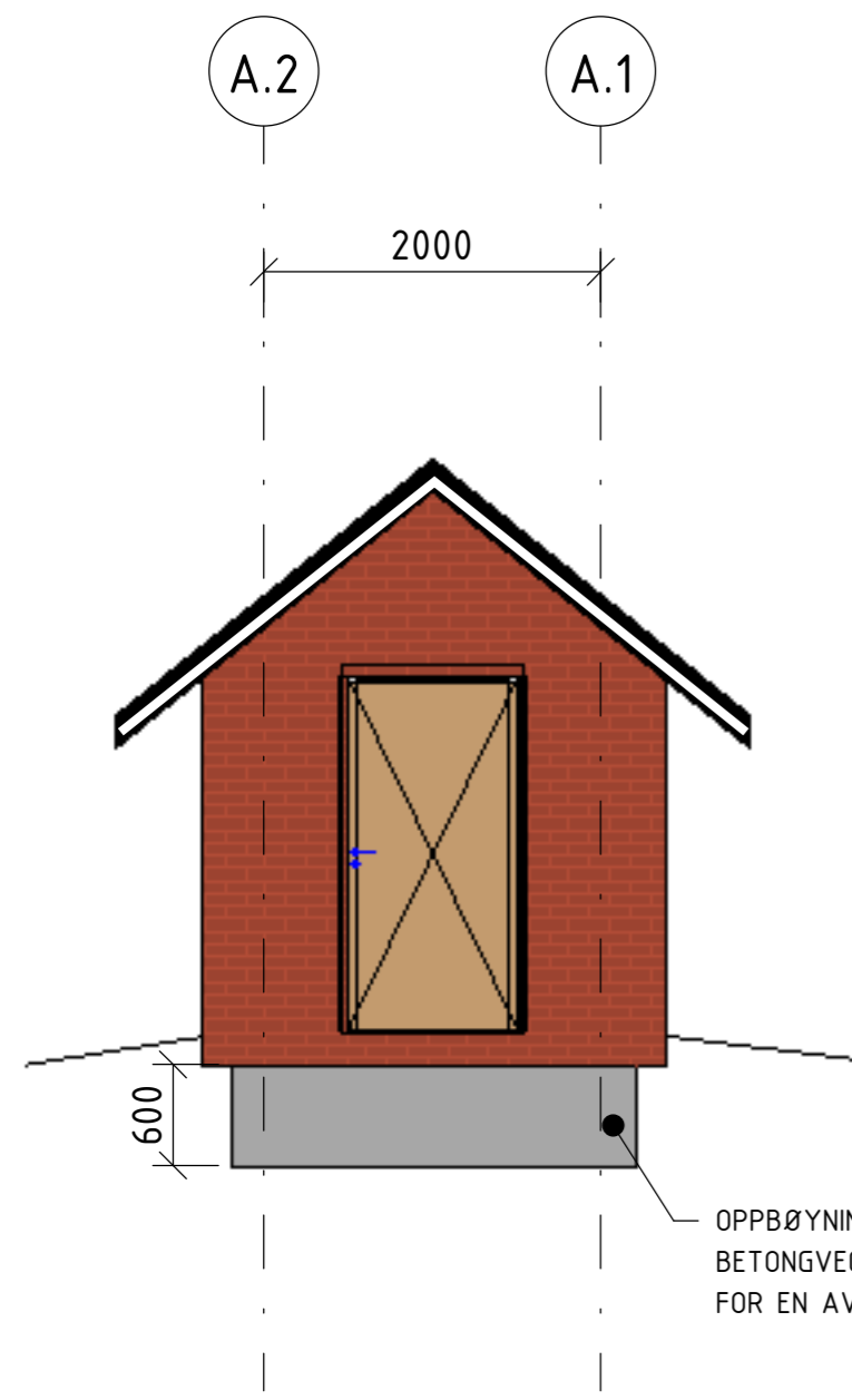
3 Fasade Nord - Brønnhus 1 : 50
