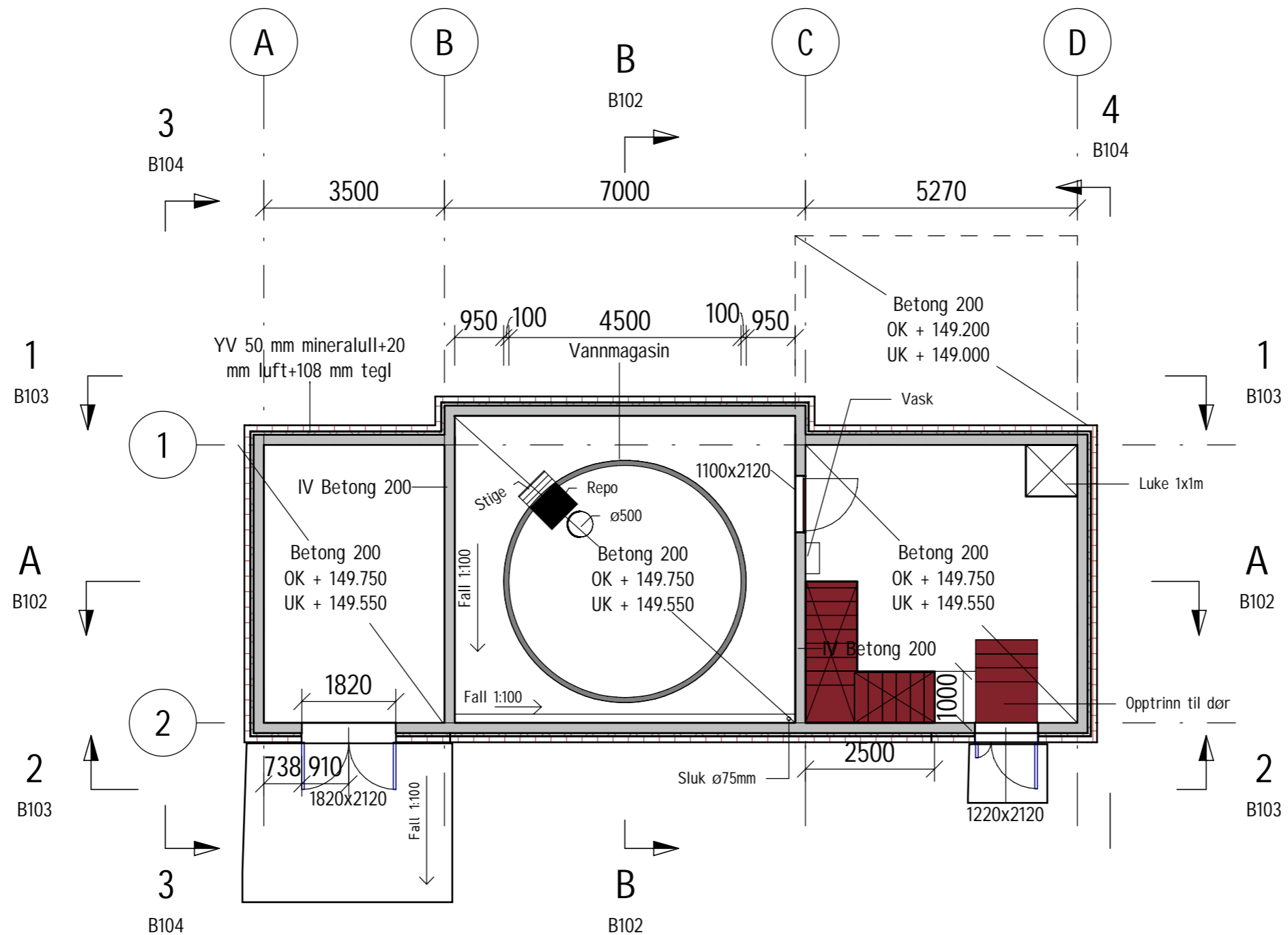
PLAN 01 FORM 1 : 100
