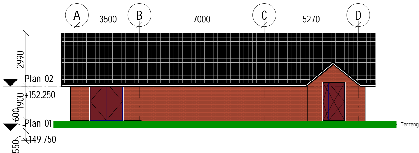
1 Fasade NORD 1 : 100
