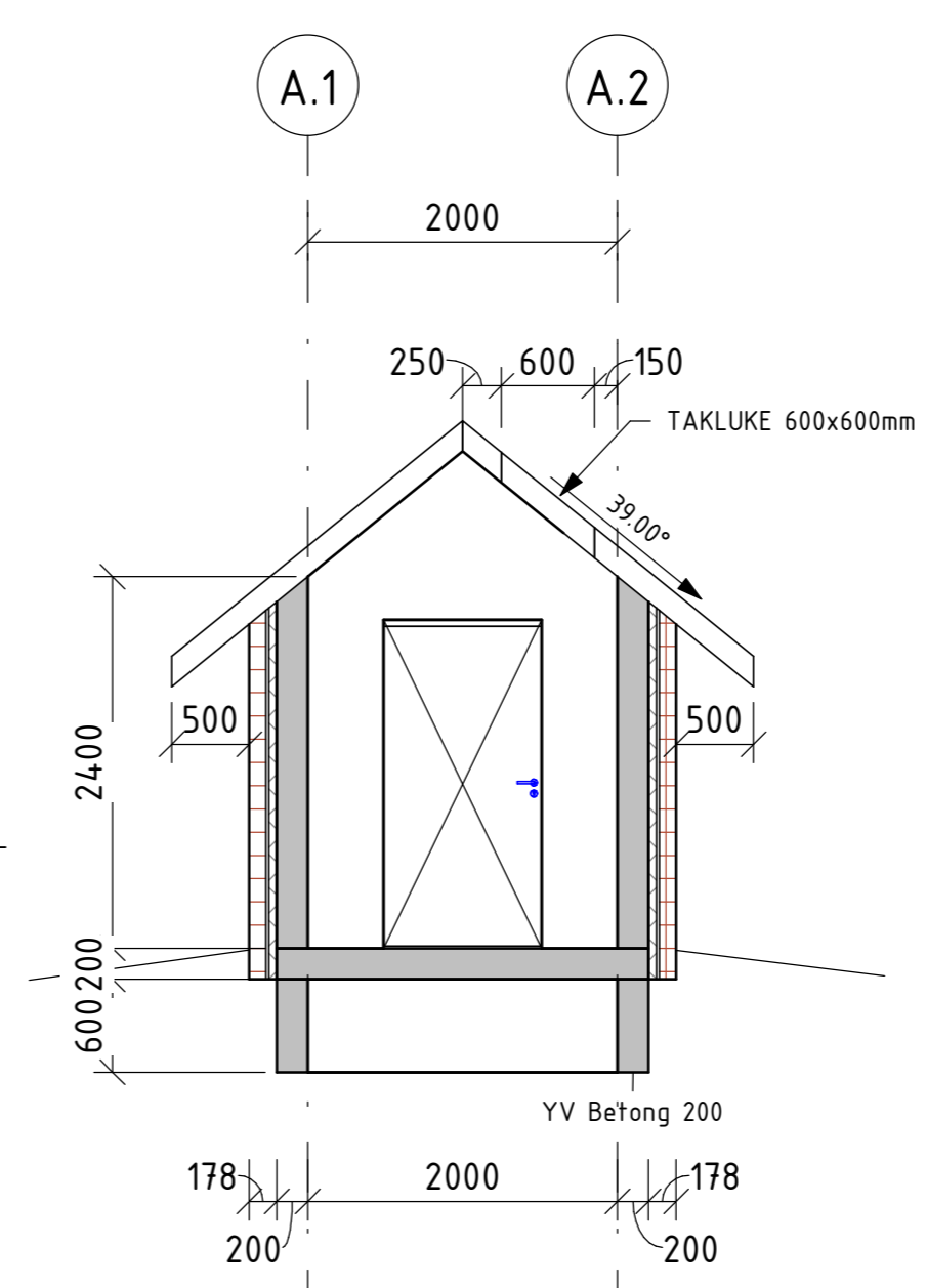
A-A Snitt - Brønnhus 1 : 50
