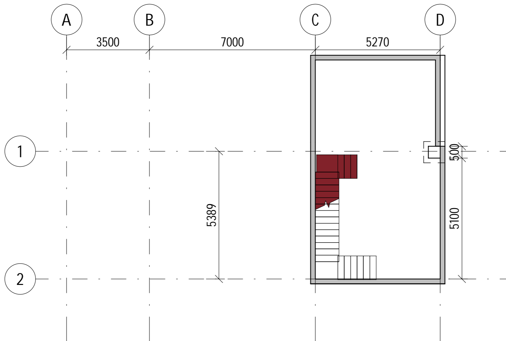
PLAN U1 FORM 1 : 100
