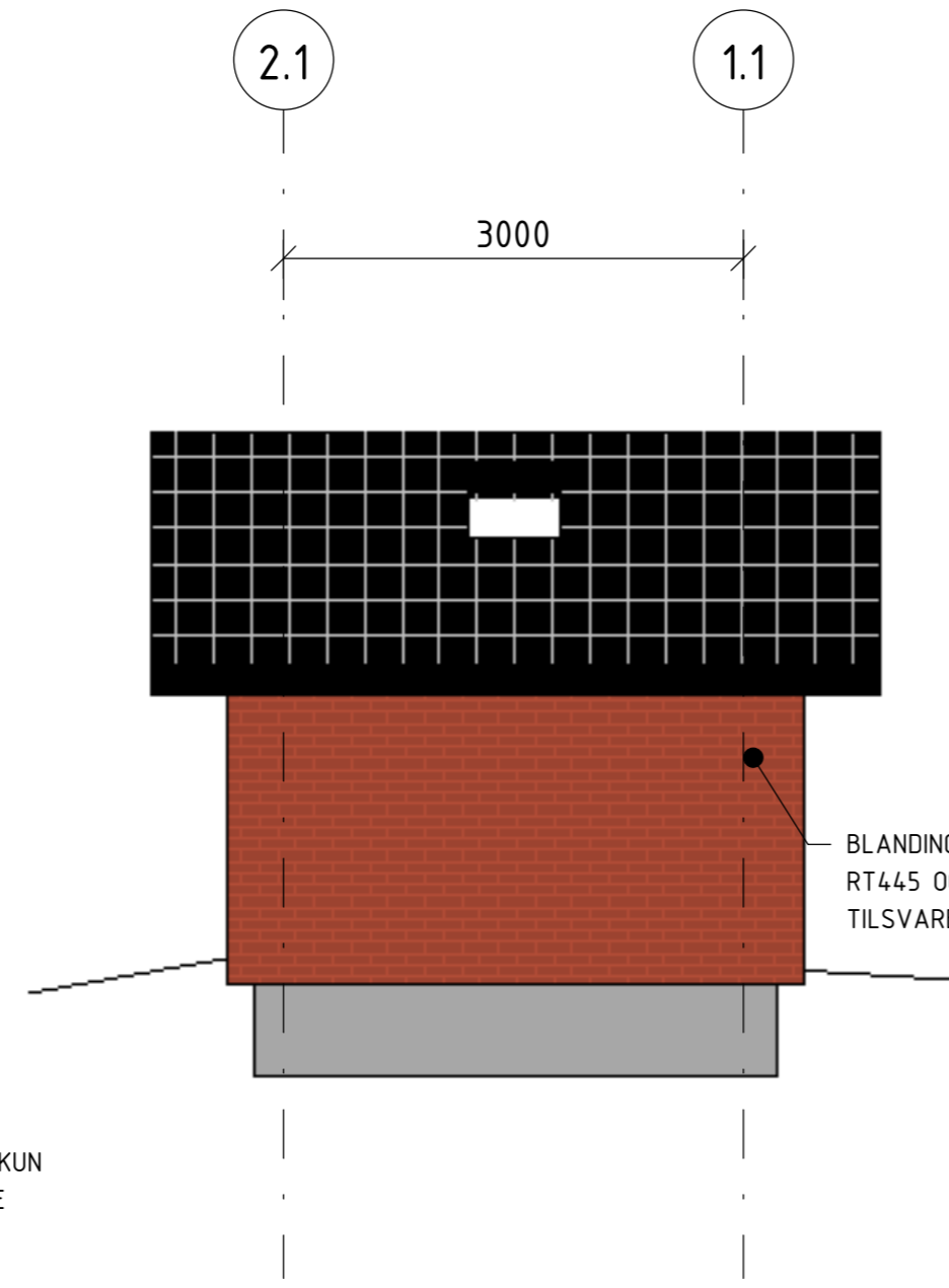
4 Fasade Øst - Brønnhus 1 : 50
