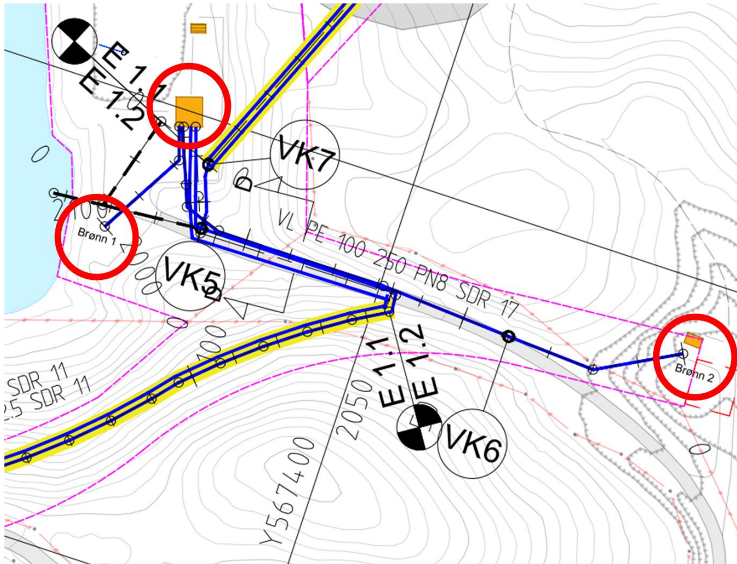
Oversiktsplan med pumpehus og brønner 23.06.2023
