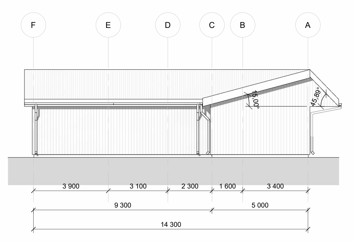
Fasade Nord 1: 100
