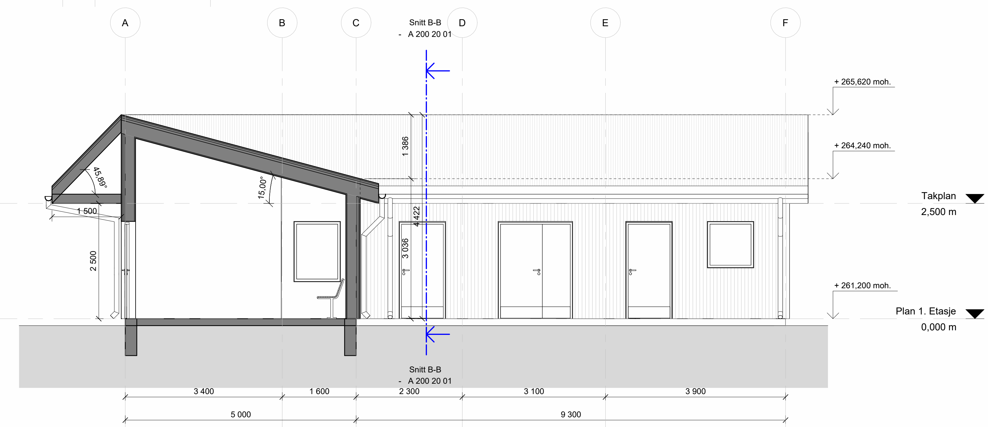
Snitt A-A 1: 50
