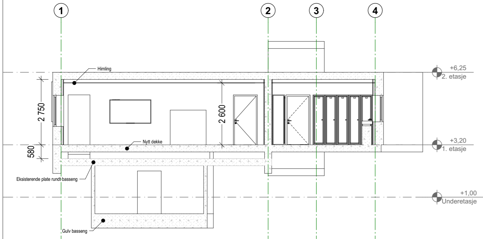
1:100 Snitt B
