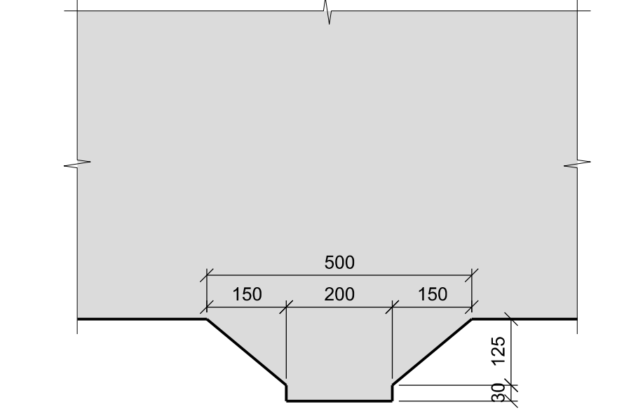
Detalj sokkel - Oppriss 1:10
