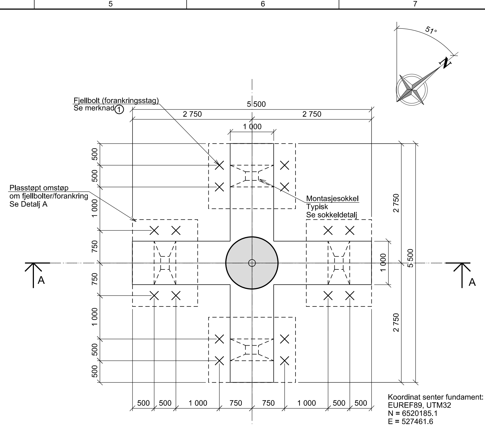
SNITT B-B. PLAN. 1:50
