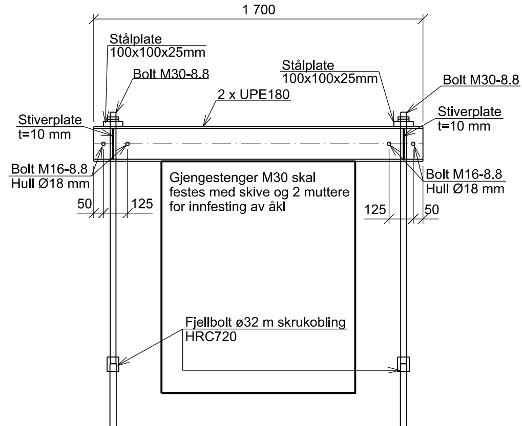
Detalj B-1 Åk - UPE 180 1:20
