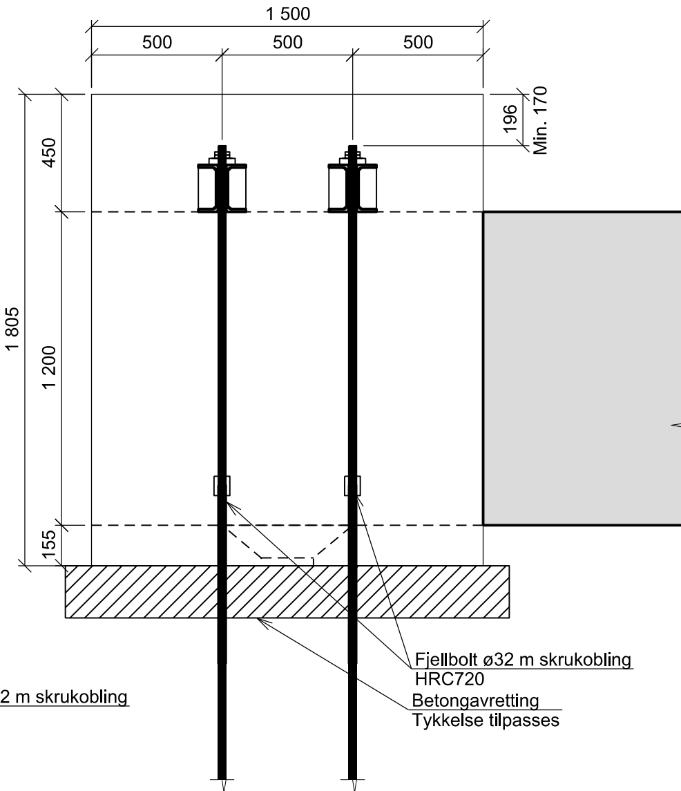
Detalj A - Omstøp ÅK og fjellbolter 1:20
