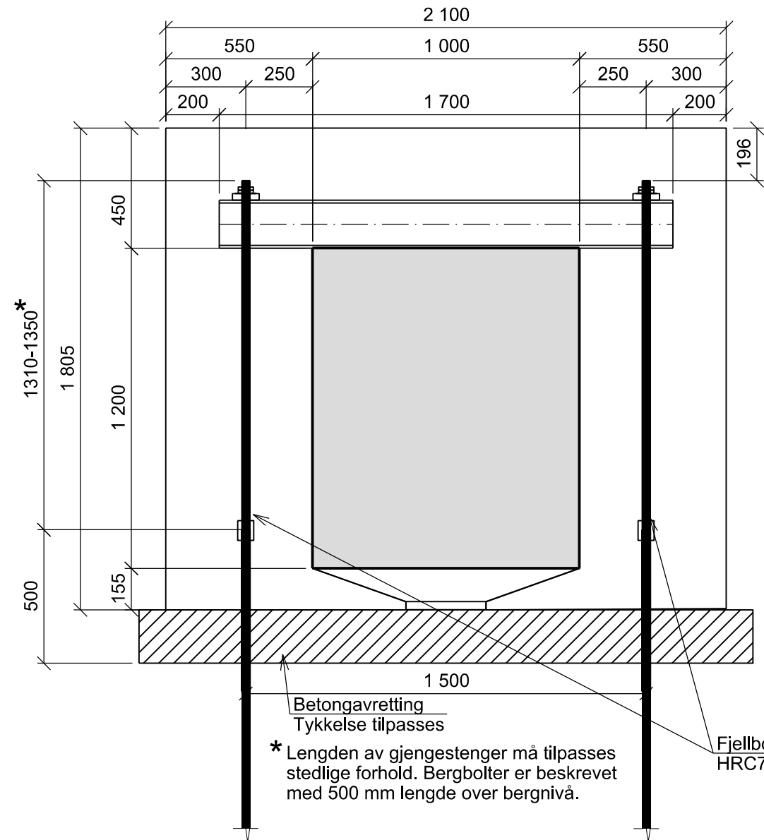
Detalj A - Omstøp ÅK og fjellbolter 1:20
