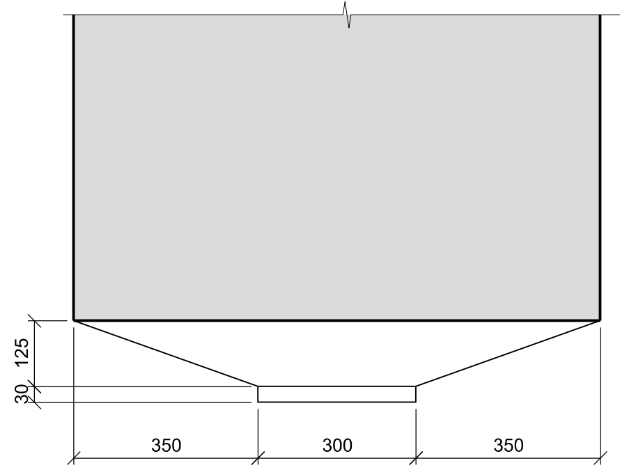
Detalj sokkel - Oppriss 1:10
