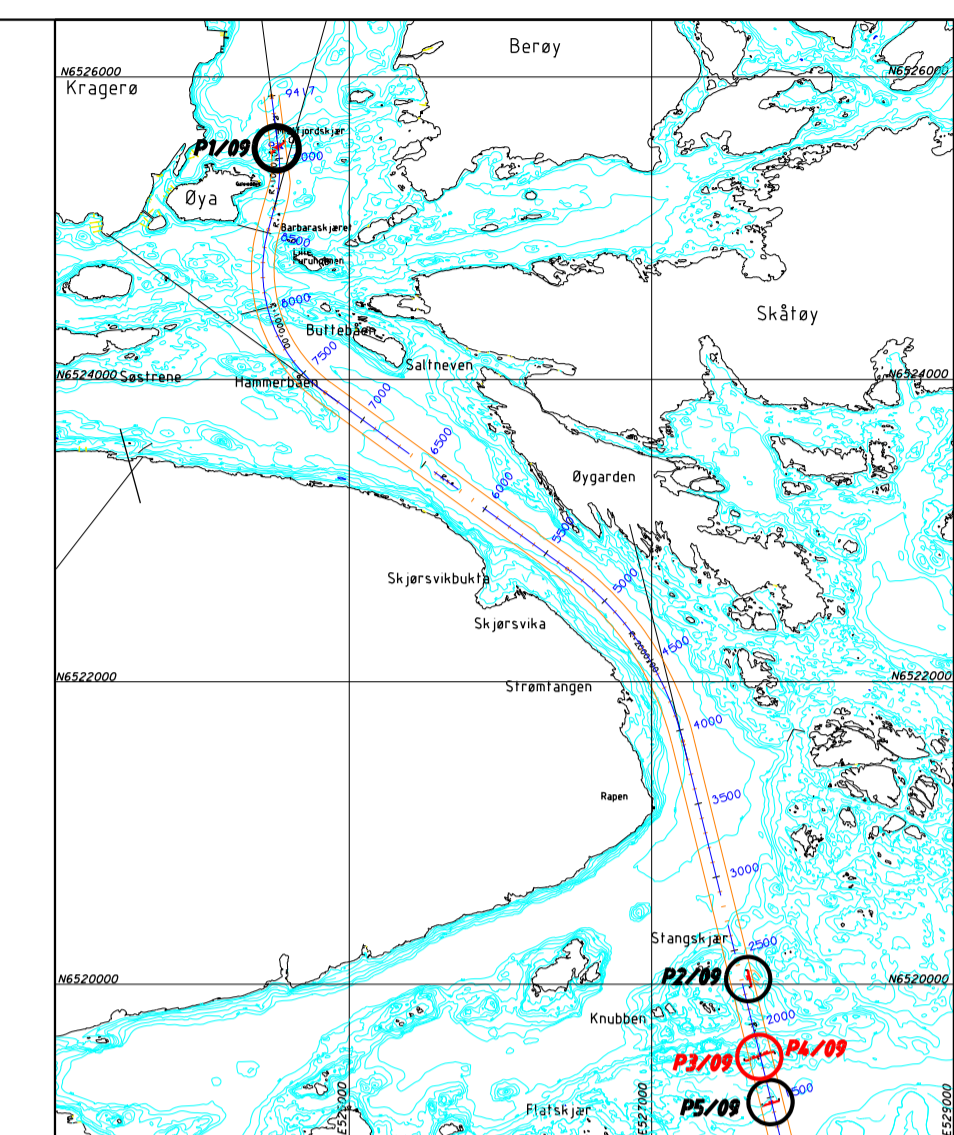
FARLED KRAGERØ Oversiktskart i refraksjonsseismiske målinger P1-P5/09
