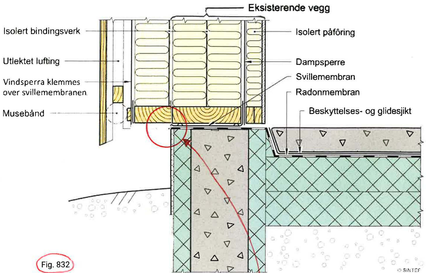
Eksempel på tilslutning til ringmur med gulv på grunnen
