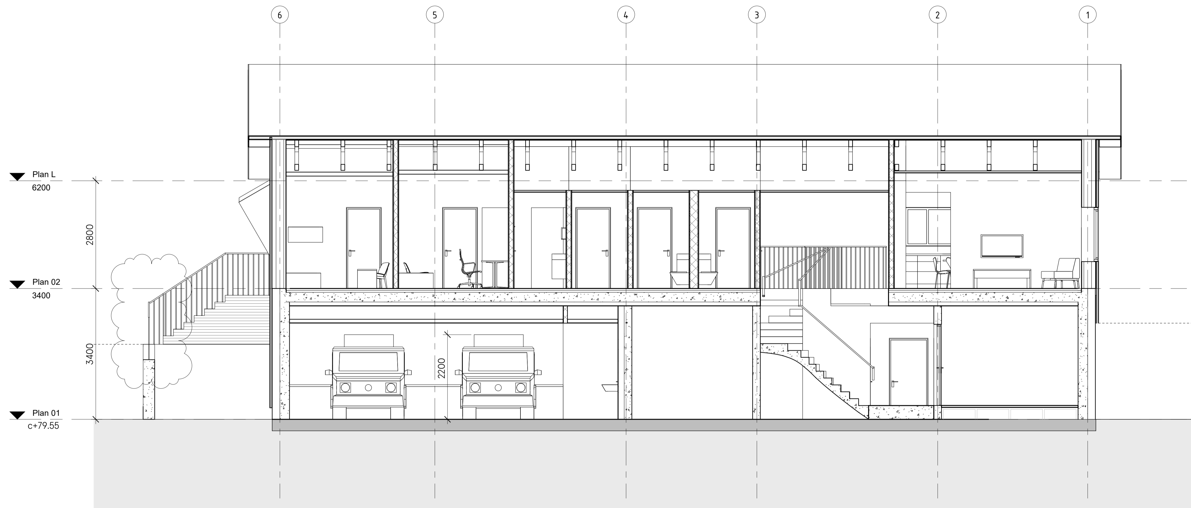
Langsnitt C 1 : 50
