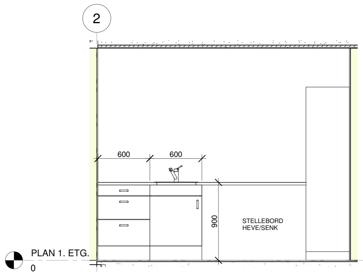
OPPRISS INNREDNING ROM A 106 1 : 25
