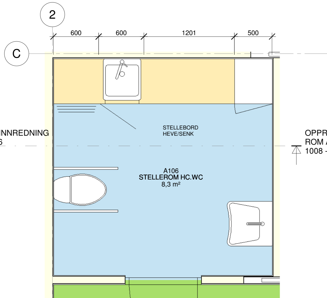
PLAN 1. ETG. -INNREDNING ROM A 106 1 : 25
