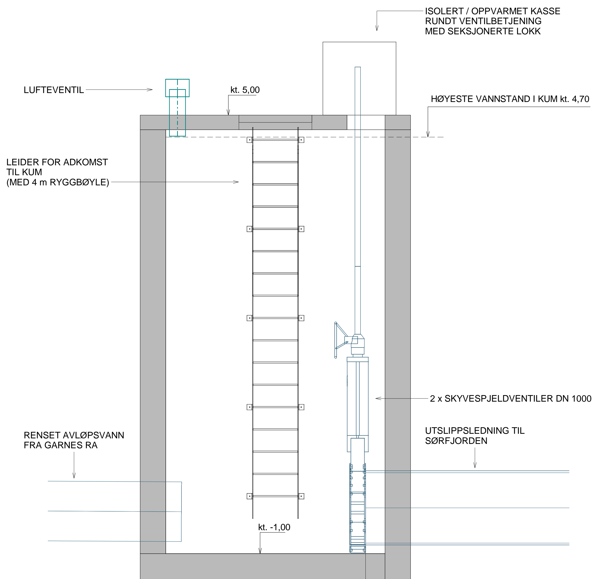
SNITT 1-1 RENSET AVLØPSVANN
