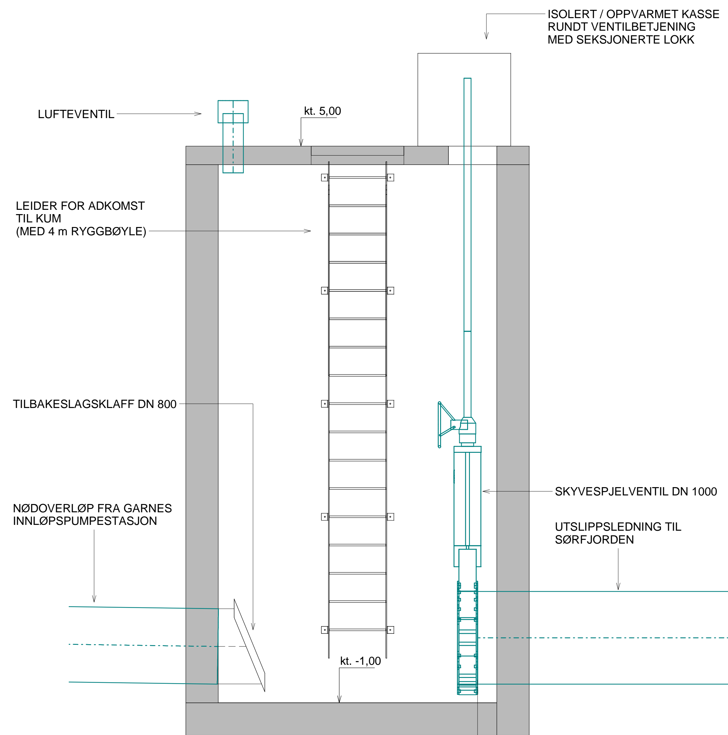
SNITT 2-2 NØDOVERLØP
