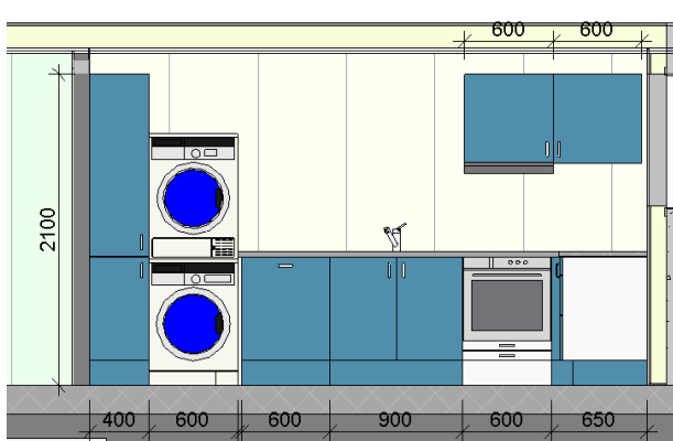
Oppriss kjøkken 1
