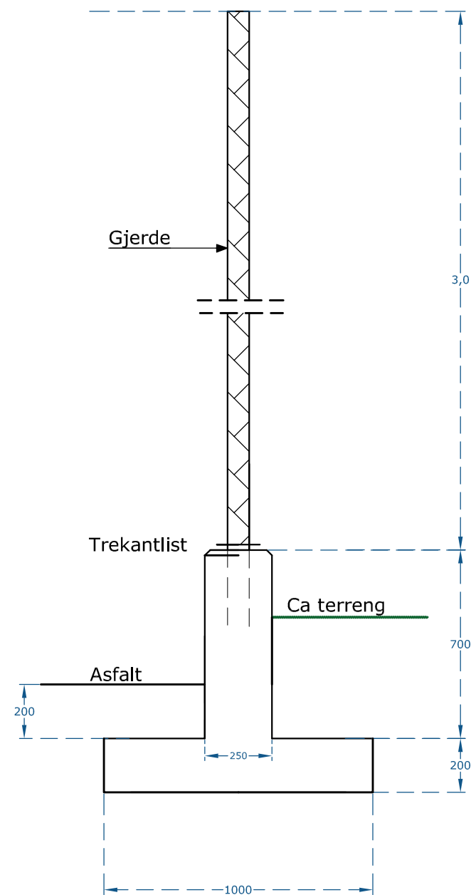
SNITT GENERELL MUR M 1:20
