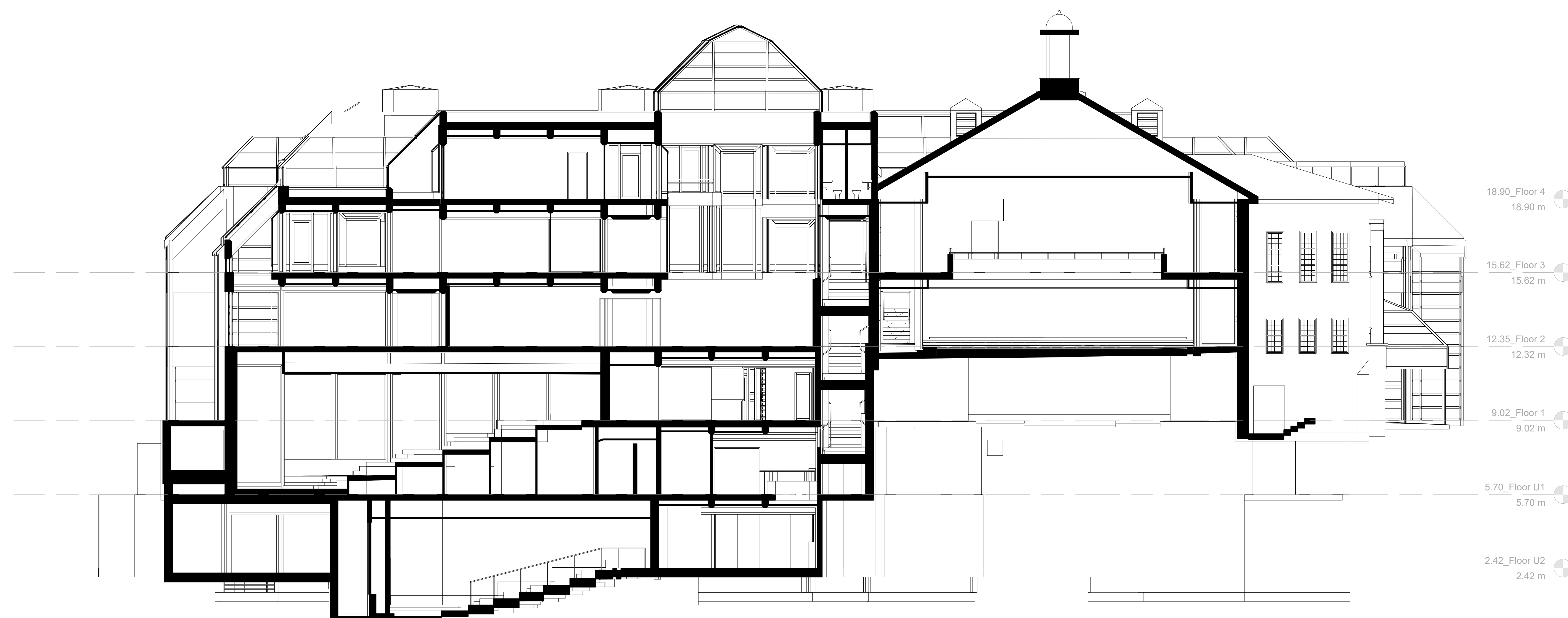
② Section 4 1 : 100
