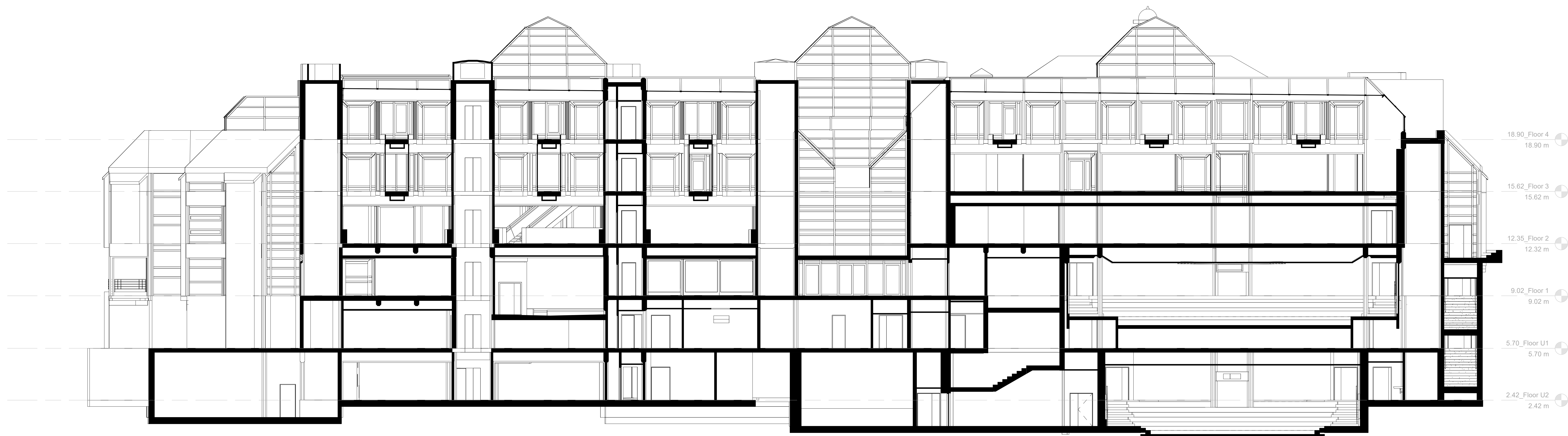
① Section 3 1 : 100
