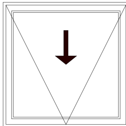
Vindu type V4 Dimensjon: Bredde ca 1,1 m, høyde ca 1,1 m Type vindu: 1-fags 1-rams vindu, trekarm Behandling: Malt tre Hengsling: Utadslående horisontalt glidehengslet Sprosser: Ingen Andre krav: (Rw+ Ctr) \geq 36 dB
