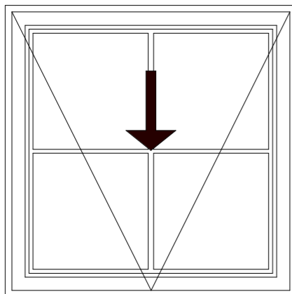
Vindu type V3 Dimensjon: Bredde ca 1,1 m, høyde ca 1,1 m Type vindu: 1-fags 1-rams vindu, trekarm Behandling: Malt tre Hengsling: Utadslående horisontalt glidehengslet Sprosser: Løse utenpåliggende Andre krav: (Rw+ Ctr) \geq 33 dB
