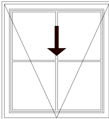
Vindu type V2 Dimensjon: Bredde ca 1,1 m, høyde ca 1,2 m Type vindu: 1-fags 1-rams vindu, trekarm Behandling: Malt tre Hengsling: Utadslående horisontalt glidehengslet Sprosser: Løse utenpåliggende Andre krav: (Rw+ Ctr) \geq 32 dB
