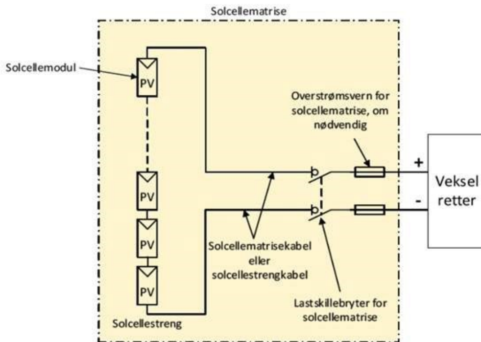
Figur 5 Prinsippskisse for én solcellestreng tilkoblet én inngang til en vekselretter. Det foreslås å ha 20-21 solcellemoduler i serie for å treffe vekselretterens spenningsvindu. Kilde: NEK400 2018.
