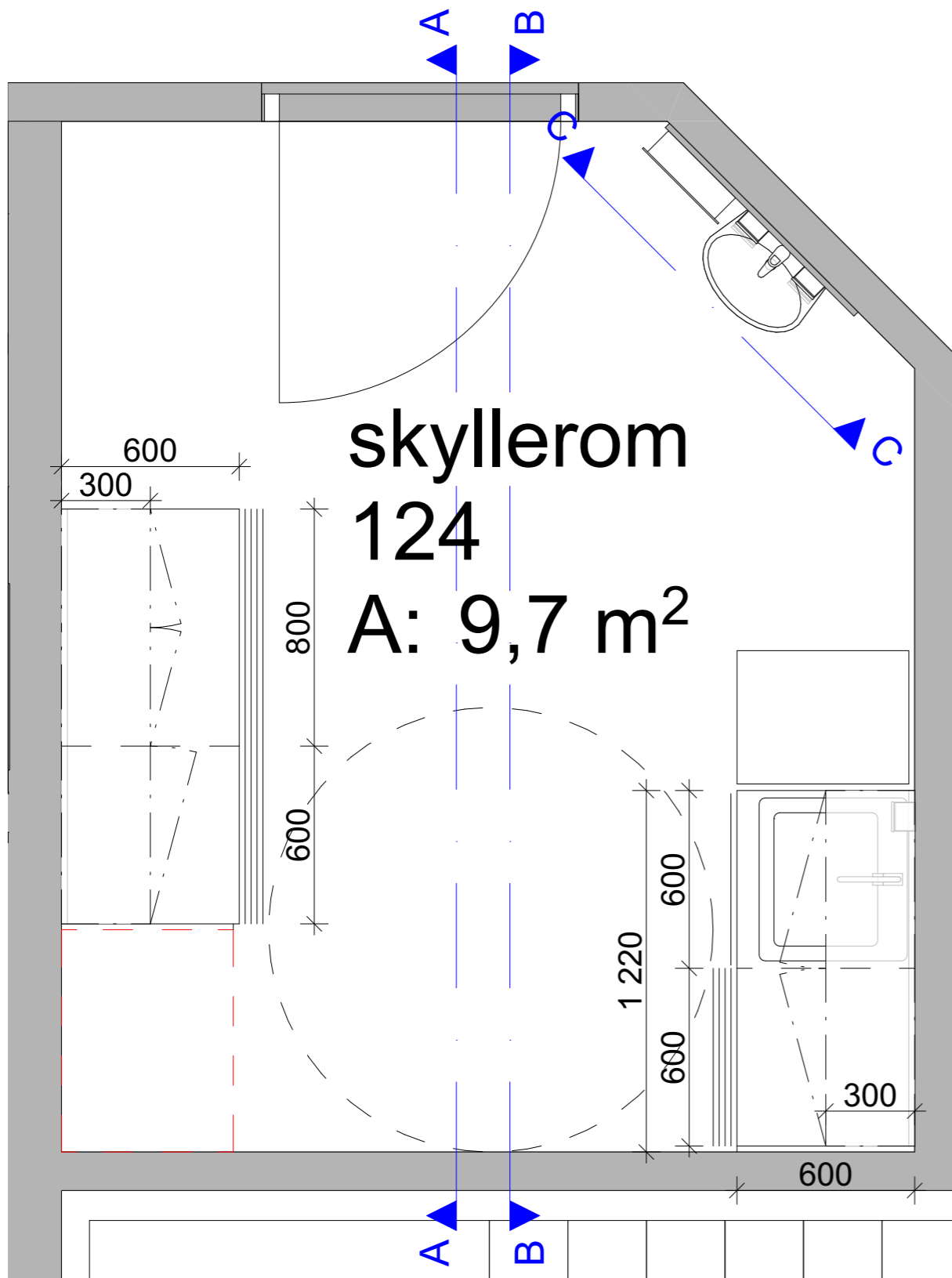
PLAN 1:20
