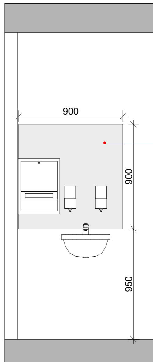
OPPRISS C-C 1:20
