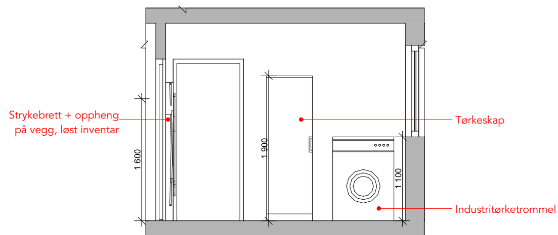
OPPRISS A-A 1:50
