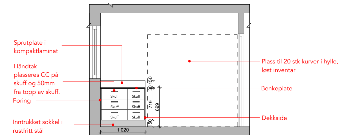
OPPRISS B-B 1:50
