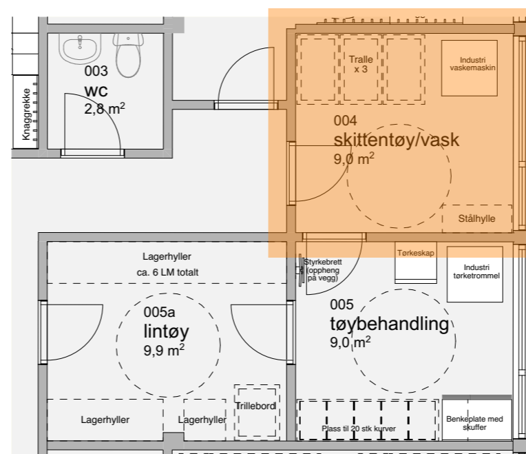
PLANUTSNITT
