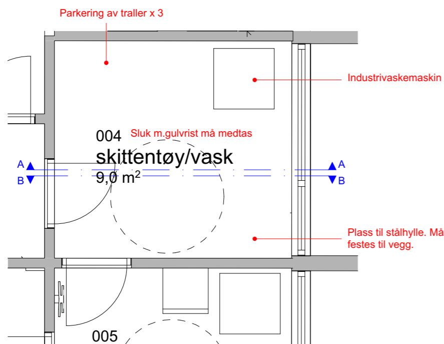
PLAN 1:50
