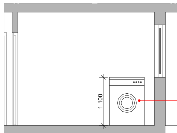
OPPRISS A-A 1:50
