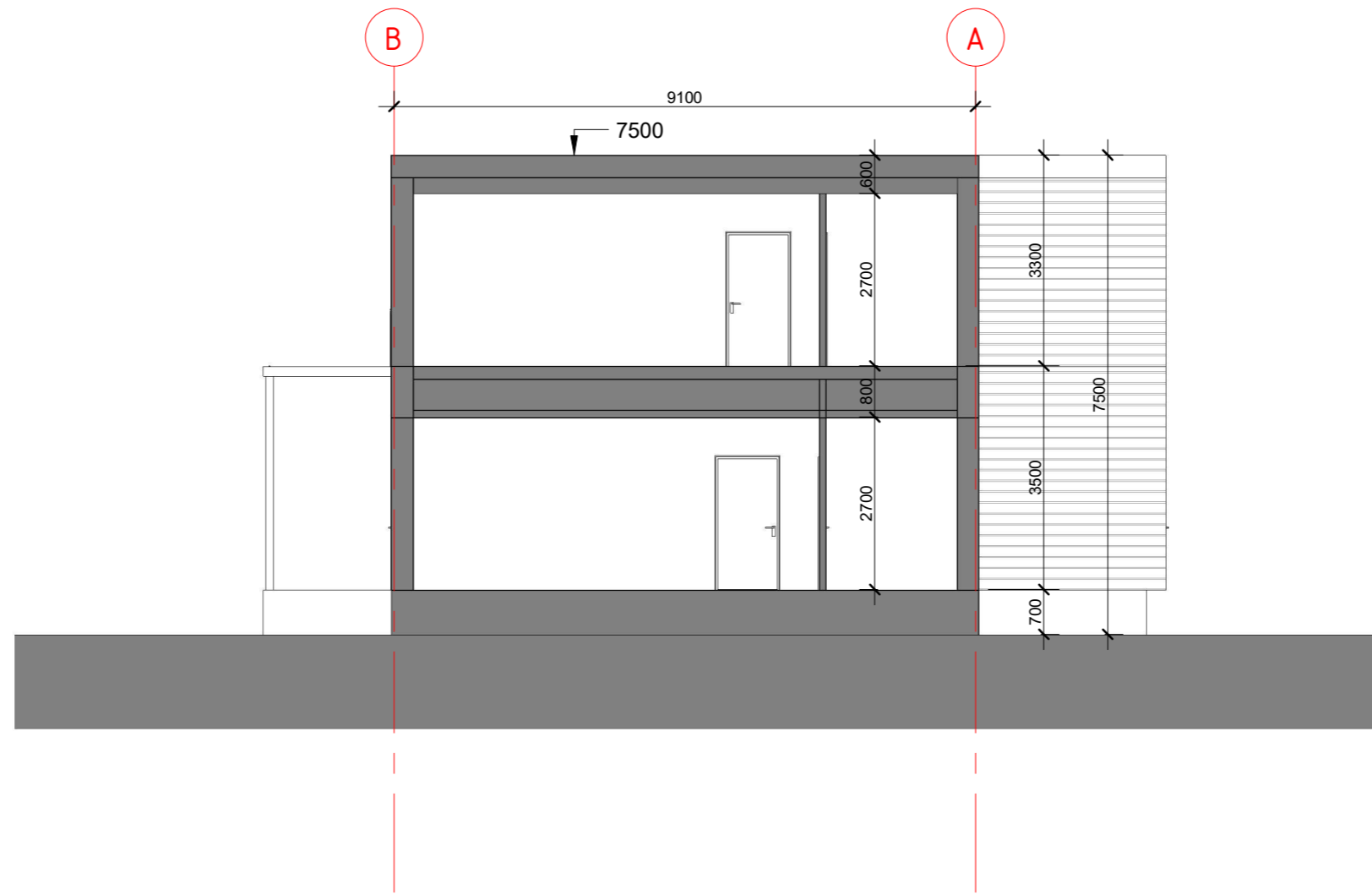
Snitt 1 1 : 100
