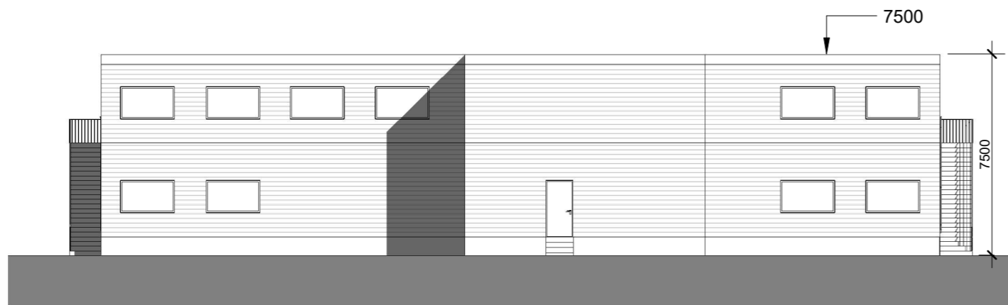
Fasade Nord 1 : 200
