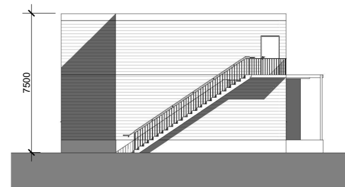
Fasade Vest 1 : 200
