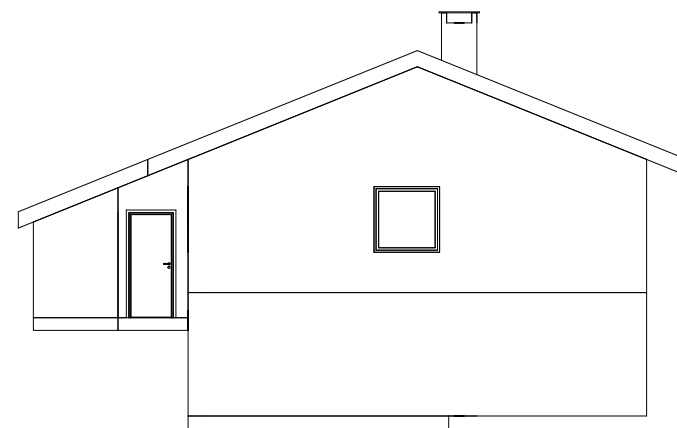
Fasade 4 1 : 150
