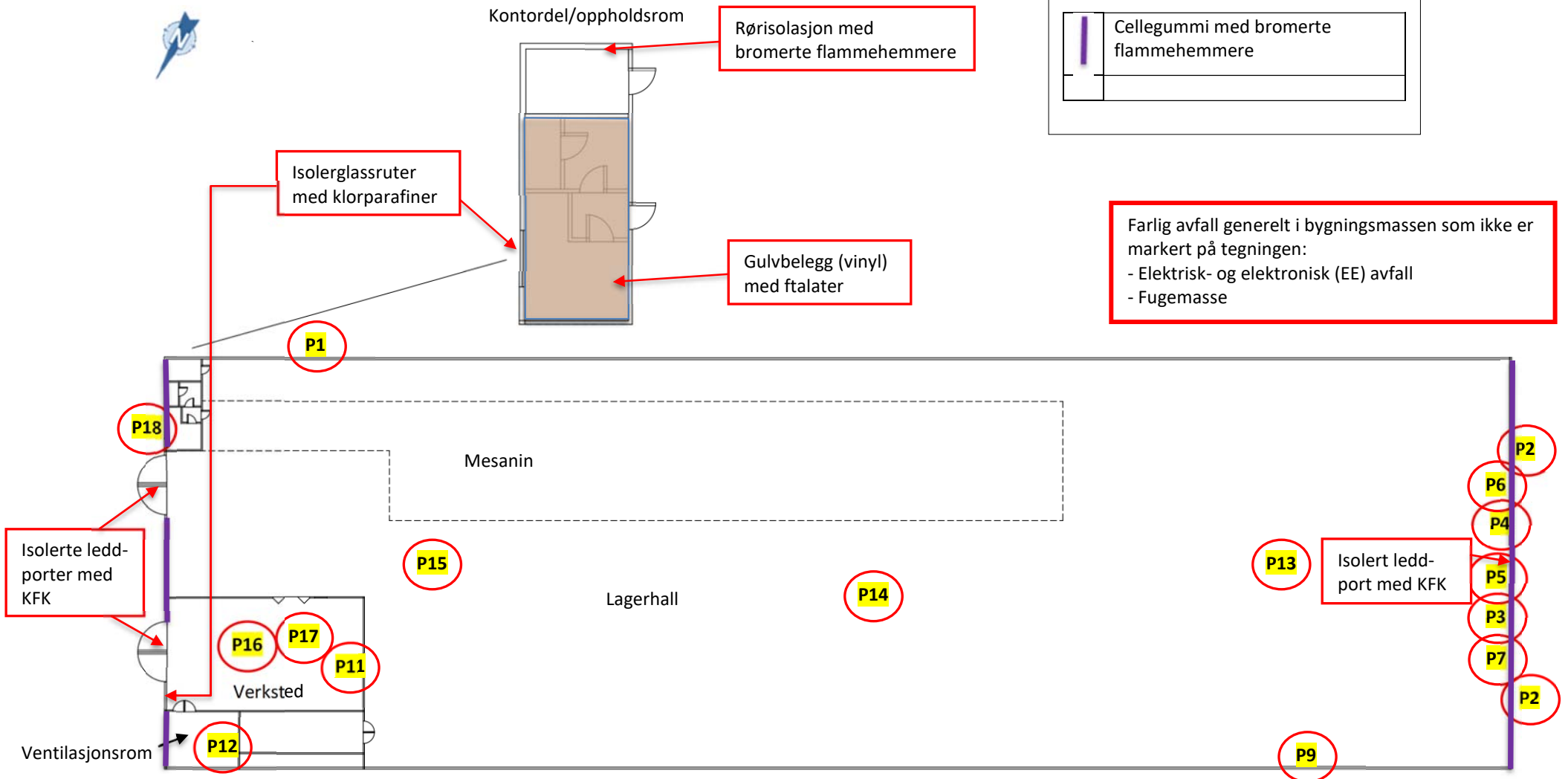
Figur 10: Plantegning med prøvetakingspunkter (P1–P7, P9 og P11–P18) og registreringer av farlig avfall i første etasje i lagerhallen, verkstedet, ventilasjonsrommet og kontordelen. Kilde: Tegning nr. VSD/BA 1201030025 COB Hall, mottatt fra Forsvarsbygg.
