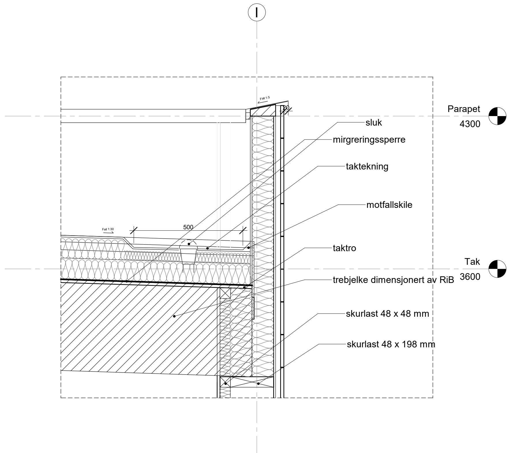
Parapet detalj 1 : 10
