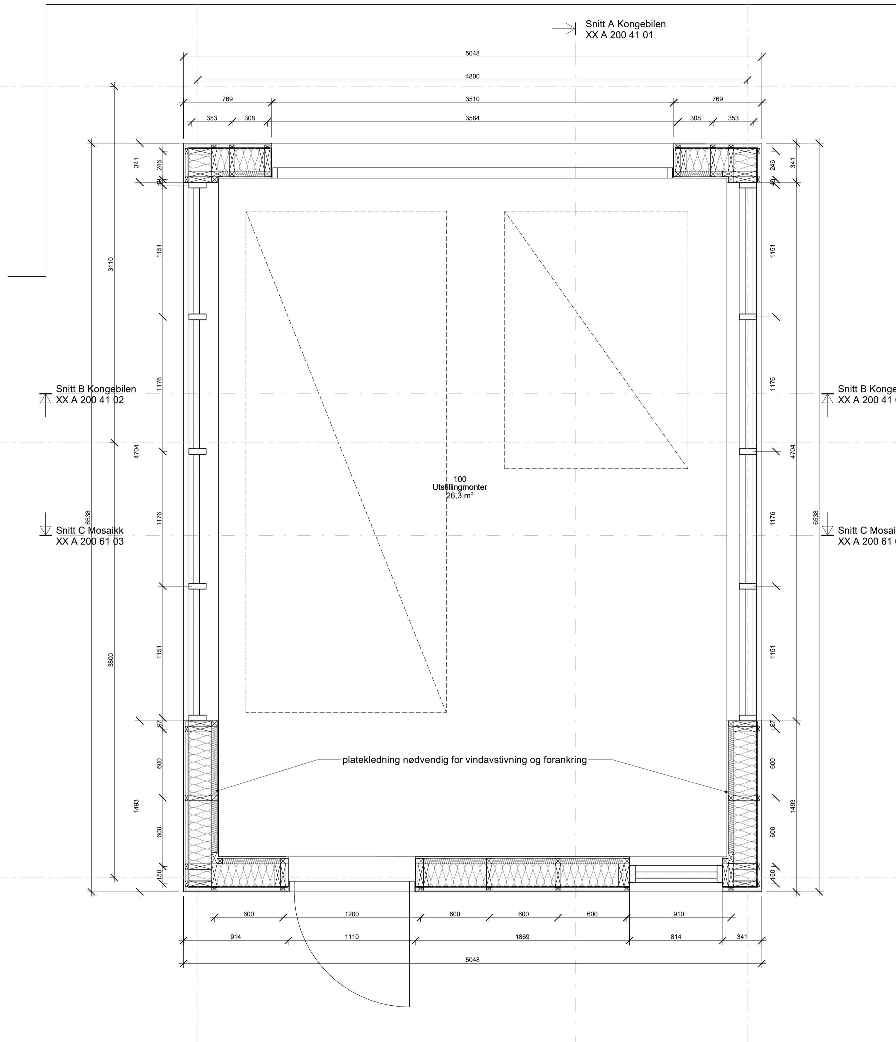
Kongebilen 1. etasje 1 : 20
